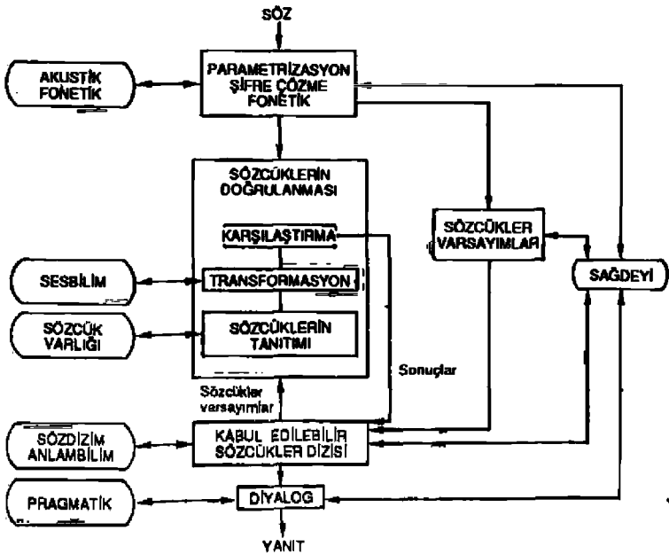
Şekil 16.- Sözüñ anlaşılması sisteminin bileşenleri.
