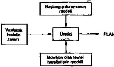
Şekil 18.- Bir plan üreticisinin yapısı
