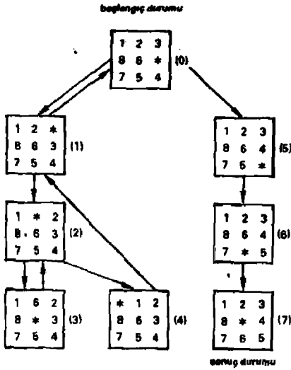
Şekil 4.- 3 x 3 oyununun derinlemesine çözümü.
