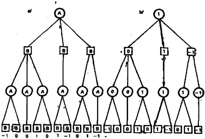
Şekil 7. Oyun ağacı ve "minimax" algoritma
