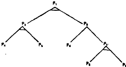
Şekil 1.- Bir VE-VEYA problem çözümleme ağacı
