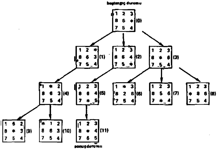
Şekil 3.- 3 x 3 oyununun enlemesine çözülmesi
