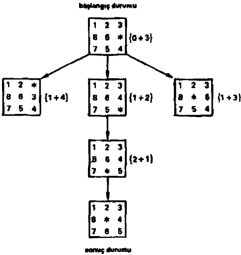
Şekil 5.- 3 x 3 oyununun düzenli araştırma ile çözülmesi
