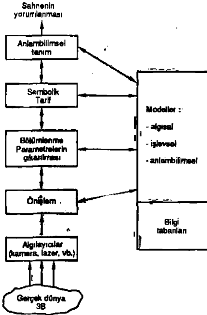
Şekil 19- Bir bilgisayarla görme sisteminin genel yapısı.
