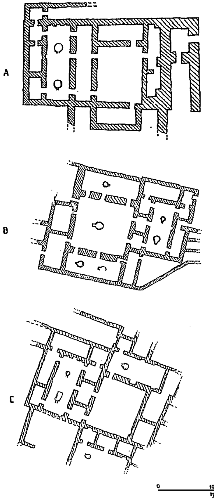
Betim 57. Son Uruk dönemi koloni yerleşmelerindeki evlerin tipolojisi. A: Hassek Höyük (Behm-Blancke [yay. haz.] 1984'ten); B: Habuba Kabira (Strommenger 1980'den); C: Cebel Aruda (van Driel Murray 1983'ten).
