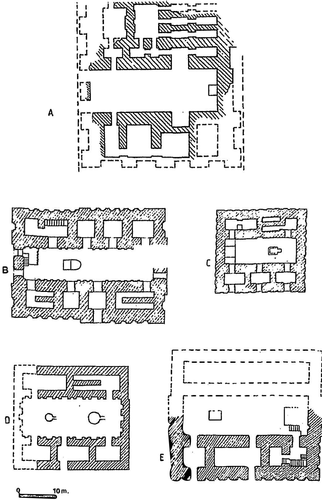
Betim 61. Son Uruk dönemi tapınakları. A: 'Gözler Tapınağı' (Mallowan 1947'den); B: Uruk'taki 'Beyaz Tapınak' (Schmidt 1972'den); C: Cebel Aruda'daki 'Kırmızı Tapınak' (van Driel, van Driel Murray 1983'ten); D: Tell Kânnas'taki 'Kuzey Tapınağı' (Finet 1979'dan); E: Ukeyr Höyüğü'ndeki 'Boyalı Tapınak' (Lloyd 1943'ten).
