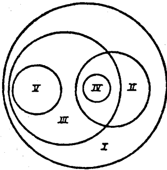
(Şekil 1a) Altküme ilişkileri
