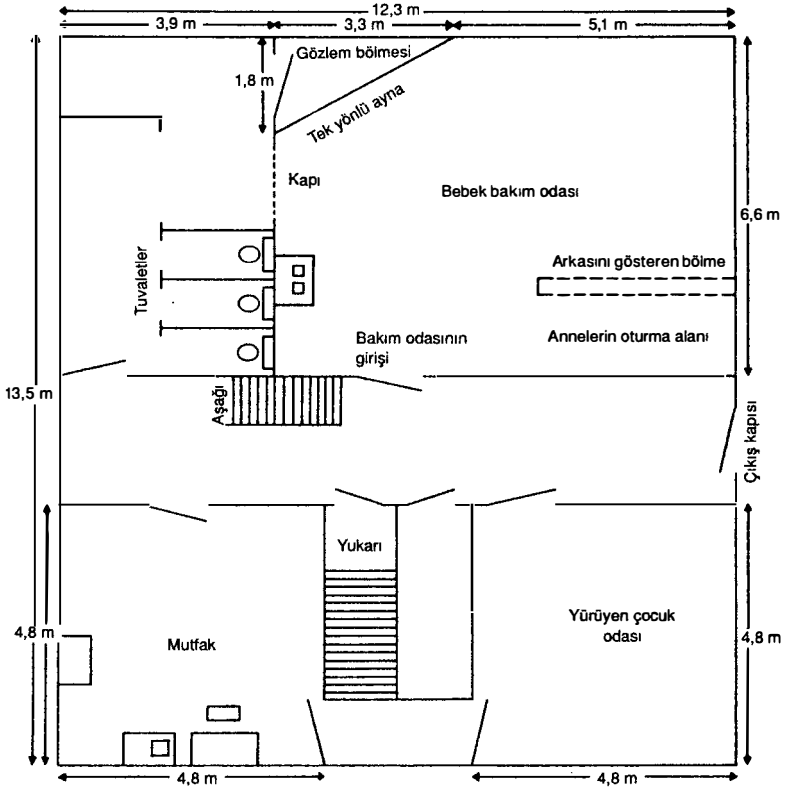
ŞEKİL 2 KAT PLANI. İLK DÜZENLEME
