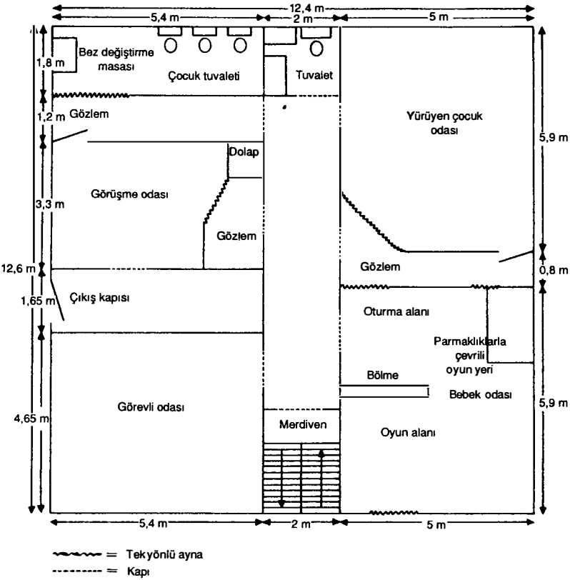
ŞEKİL 3 KAT PLANI. İKİNCİ DÜZENLEME
