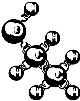
Şekil 3. Atomların halka ve kancalarla birbirlerine bağlanması.
