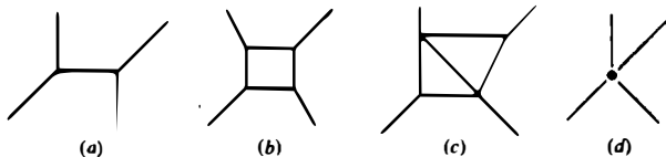
Şekil 24. (a) En basit parçacık değiş tokuş süreci. Bu tür bir diyagramda kuantum mekaniği en az etkiyi gösterir. (b) Tek bir kapalı halkadaki çoklu parçacık değiş tokuşu. (c) İki halka diyagramı. Kuantum kütleçekiminde, (d)'de gösterilen sonsuz etkileşim hesaba katıldığında, bu değiş tokuşların etkisi sonlu olur. Ancak (d)'deki etkileşim (b) ya da (c)'deki köşelere konulursa karışıklıklar kontrolden çıkar.
