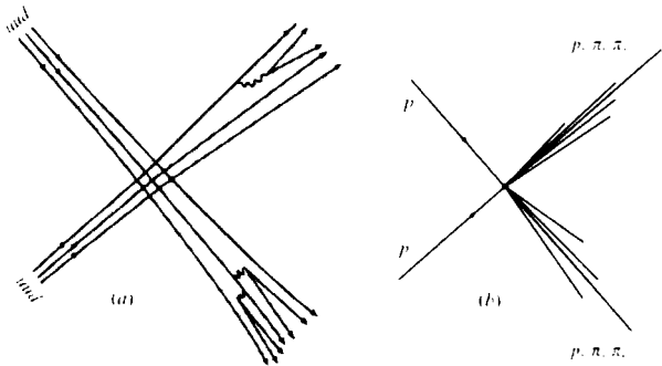
Şekil 15. (a) İki proton birbirleriyle çarpışır, ama kuarklar birbirine çarpmaz ("periferik" bir çarpışma). (b) Deneycinin çarpışma sonunda gördüğü durum.
