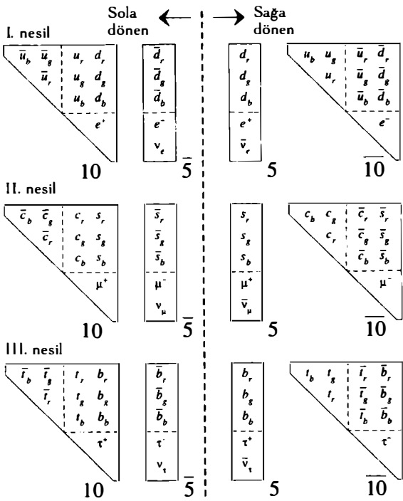
Şekil 22. Georgi-Glashow SU(5) modelindeki çoklular. Sağ ile sol elli bileşenler farklı konumlarda bulunurlar. Parçacık adlarının üstündeki çizgiler antiparçacıkları gösterir. Kuarklar R (kırmızı), G (yeşil) ve B (mavi) alt indisleriyle gösterilen üç renkte bulunurlar.
