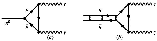
Şekil 19. \pi^0 'ın iki fotona bozunması: (a) proton-antiproton yok olması ile (b) kuark-antikuark yok olması.
