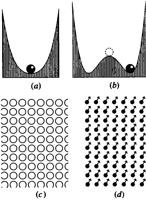
Şekil 10. Simetri ve simetrinin kendiliğinden bozulması. Simetrik denklem sisteminin kararlı ve simetrik bir çözümü olabilir (a) ya da sistem kendini simetrik olmayan bir çözümde bulabilir (b). Bir alanın simetrik bir çözümü varsa, tasvir ettiği fiziksel sistem simetrik (c). Kararlı çözüm simetrik değilse, bu fiziksel sistem de simetrik olmayan bir yapı gösterir (d).
