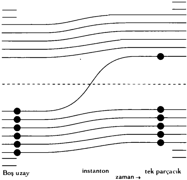
Şekil 21. Bir instanton, birlikte olduğu parçacığı sürükleyerek parçacığın bir negatif enerji konumundan bir pozitif enerji konumuna (ya da tersine) geçmesini sağlar.
