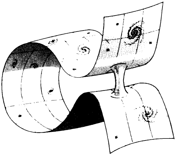
Şekil 30. Bir evrenin uzak bölgelerini birbirine bağlayabilecek bir solucan deliği.
