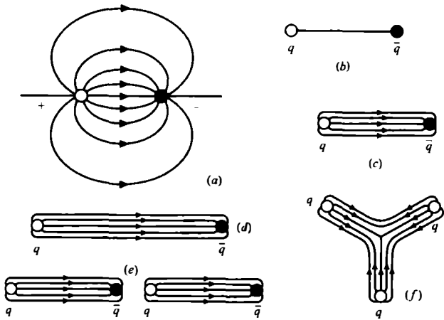
Şekil 14. (a) Maxwell'in elektromanyetik teorisinde iki yük arasındaki alan çizgileri. (b) Sicim teorisi. (c) Kuark ile bir antikuark arasındaki gluon alanı. (d) Bir kuark ile antikuark birbirinden uzaklaştırılırsa daha çok alan yaratılır ve sonunda (e) yeni bir kuark-antikuark çifti oluşur. (f) baryon. ( q =kuark, \bar{q} = antikuark).
