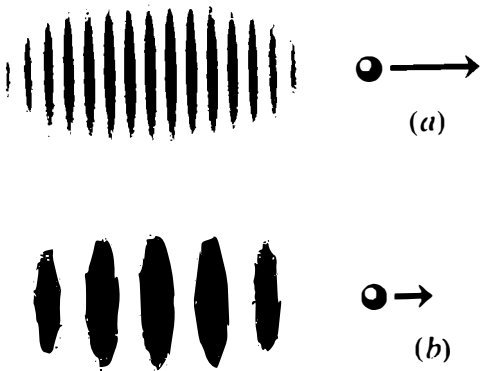
Şekil 4. Dalgalara karşılık gelen parçacıklar. Fazla enerjili parçacıklar (a), az enerjili parçacıklara (b) göre daha kısa dalga boylu ve hızlı salının yapan dalgalardan meydana gelir.
