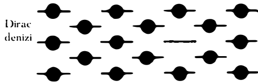
Şekil 20. Şekilde Dirac teorisine göre bir parçacık ve bir antiparçacık vardır.
