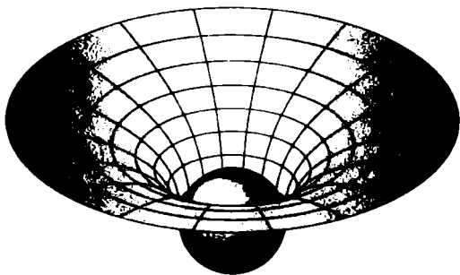
Şekil 28. Bir ressam gözüyle kara delik.
