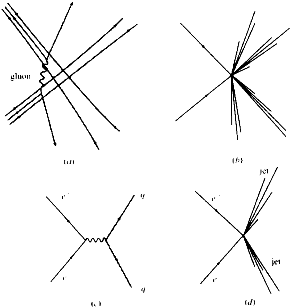
Şekil 16. (a) İki kuark birbiriyle çarpışır. (b) Deneycinin gördüğü şey: tipik bir "jet olayı". (c) e^+ + e^- \rightarrow iki kuark. (d) Bu olayın bir deneydeki görünümü.
