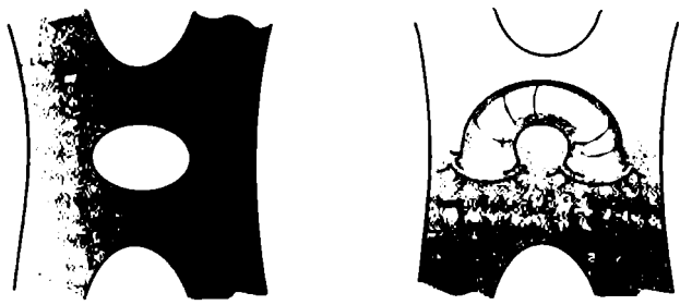
Şekil 27. Yüksek mertebeden sicim diyagramları.
