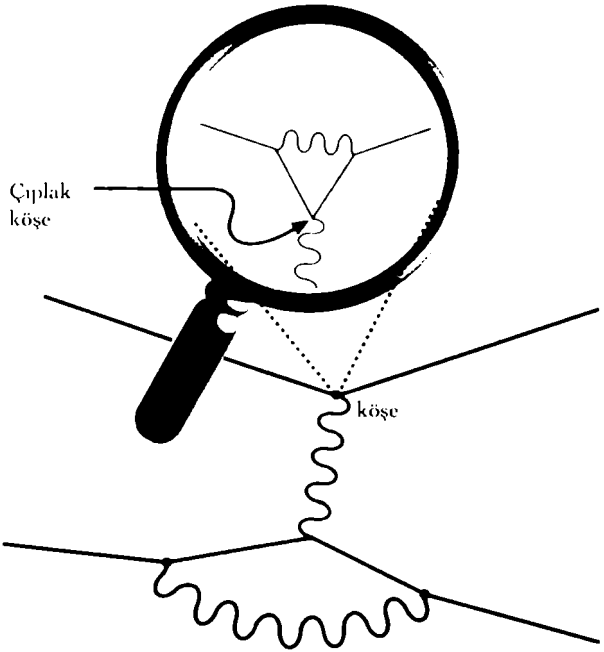
Şekil 13. Temel bir etkileşimin tanımı, büyütme ölçeğine bağlıdır.
