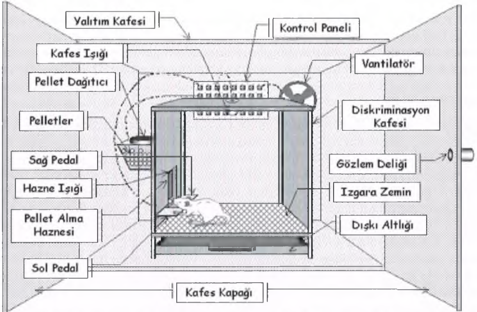
Şekil 42. Maddelerin diskriminatif (kendini ayırt ettirici) etkilerini değerlendiren düzenek (Uzbay 2004a'dan alınmıştır).
