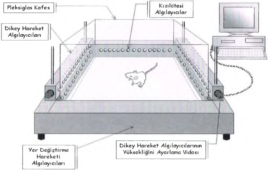
Şekil 44. Locomotor aktivite ölçüm cihazı (Uzbyay, 2004a'dan alınmıştır).
