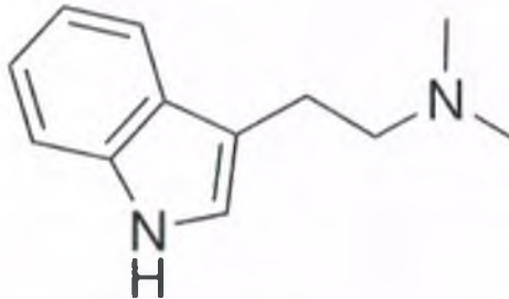
Şekil 34. Dimetiltriptamin (DMT).
