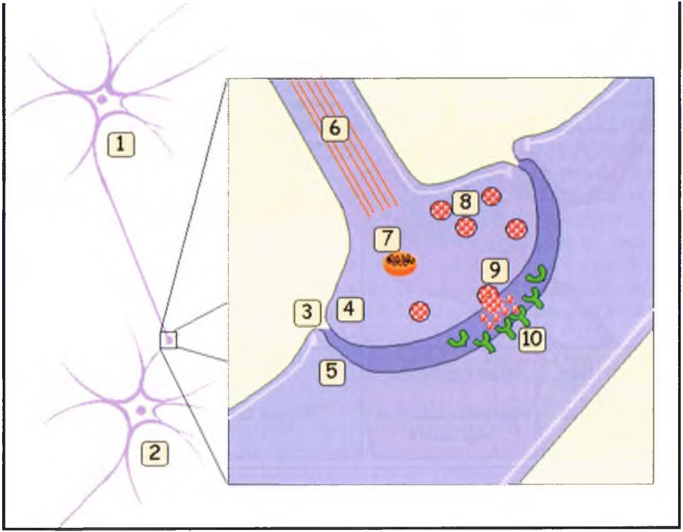
Şekil 8. Sinaps morfolojisi. 1: presinaptik nöron, 2: postsinaptik nöron, 3: sinaptik aralık, 4: presinaptik uç, 5: postsinaptik bölge, 6: mikrotübüller, 7: mitokondri, 8: nörotransmitter depolayan veziküller, 9: presinaptik vezikülden sinaps aralığına saliverilen nörotransmitter, 10: postsinaptik membranda yer alan reseptörler (Uzbay, 2004'ten alınmıştır).
