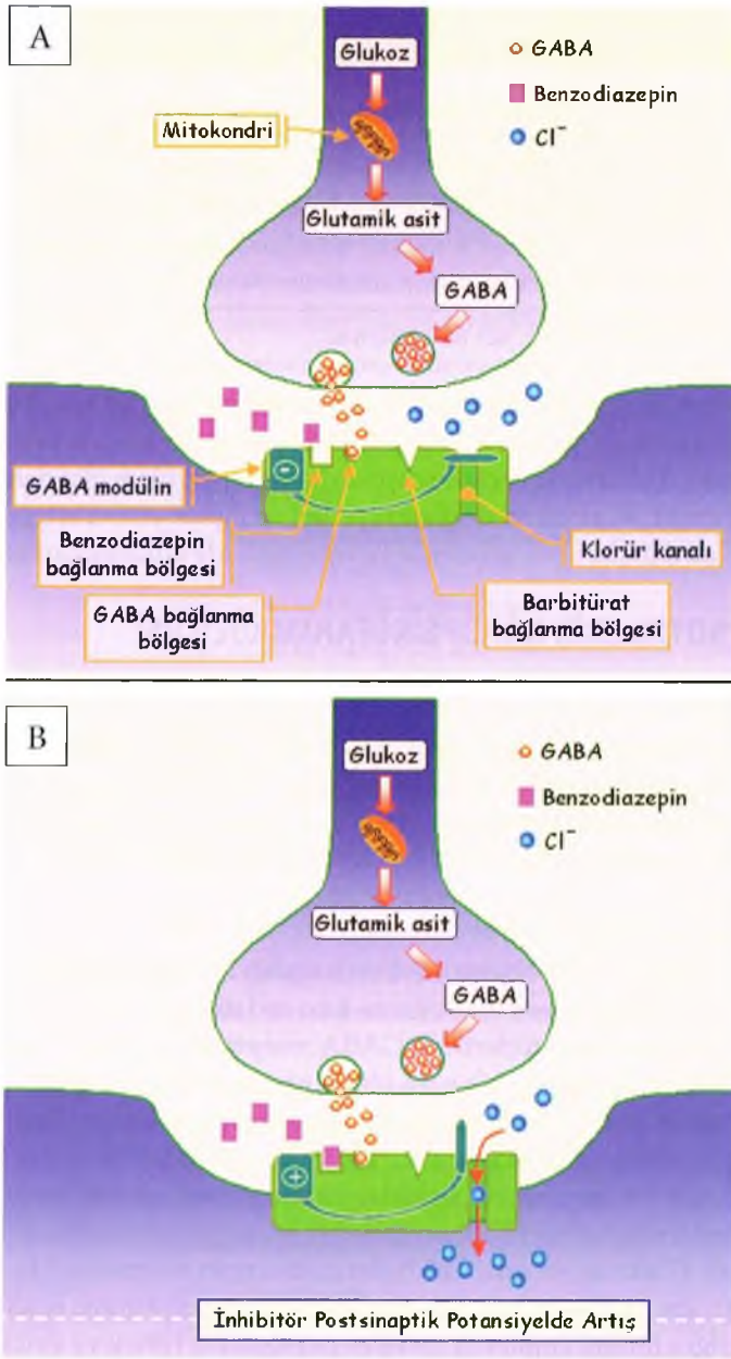
Şekil 28. GABA reseptörü-BZ reseptörü-Cl - iyonoforu (Uzbay, 2007'den alınmıştır).
