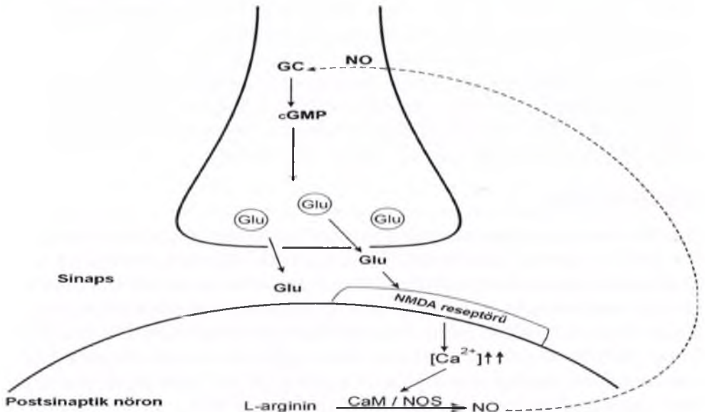
Şekil 10. Santral sinir sisteminde nitrik oksidin çalışmasını açıklayan model (GC: Guanilat siklaz, cGMP: siklik guanozin monofosfat, Glu: Glutamat) (Uzbay ve Oglesby, 2001).
