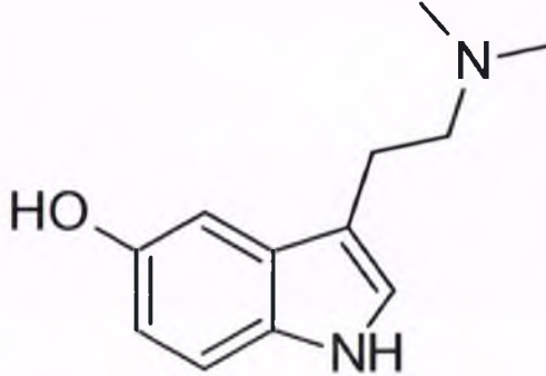
Şekil 35. Hidroksi-dimetiltriptamin (bufotenin).
