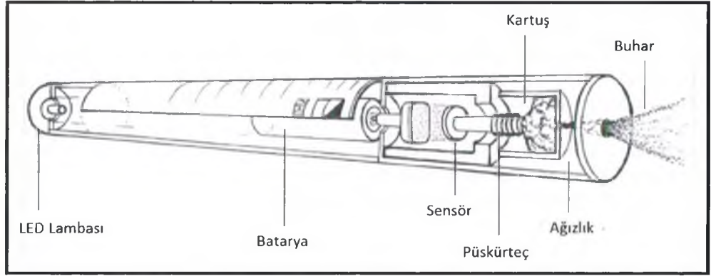
Şekil 26. Elektronik sigara şeması (Knorst ve ark., 2014).
