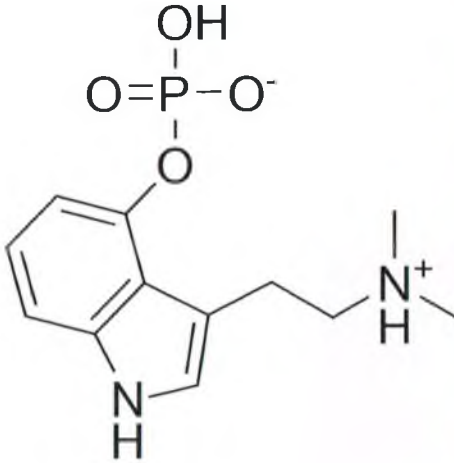
Şekil 32. Psilosibin
