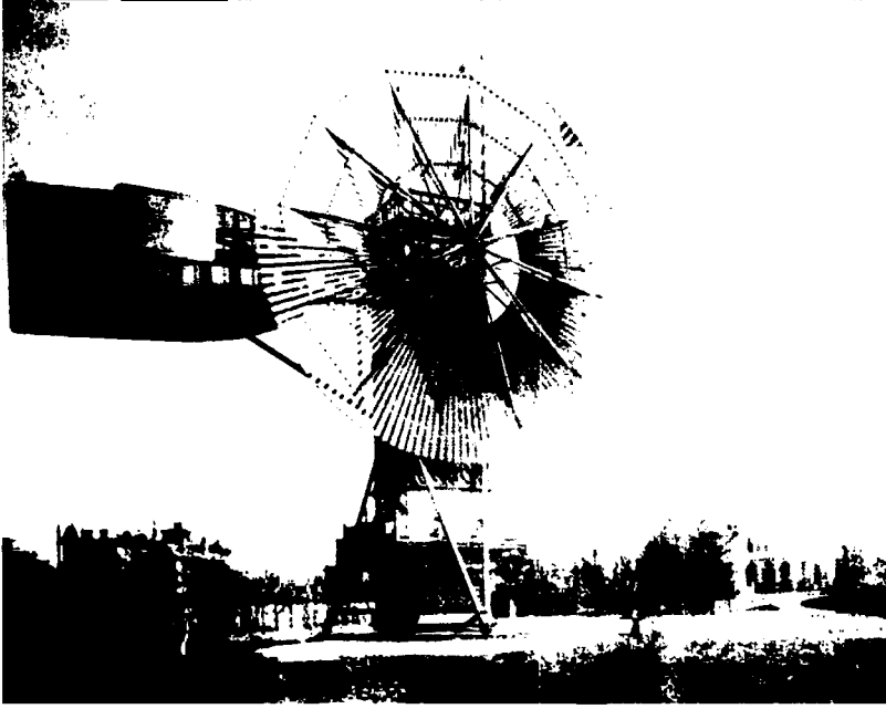
Charles Brush'ın 17 metre çapındaki, elektrik üreten yel değirmeni, inşa tarihi 1887.
