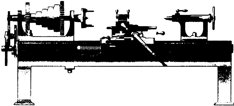
Ayna başlığı ile üzerinde çalışılan parçayı tutmaya ve döndürmeye yarayan şaft (solda); punta başlığı (sağda) ve kesme takımını taşıyan hareketli vagon (ortada).
