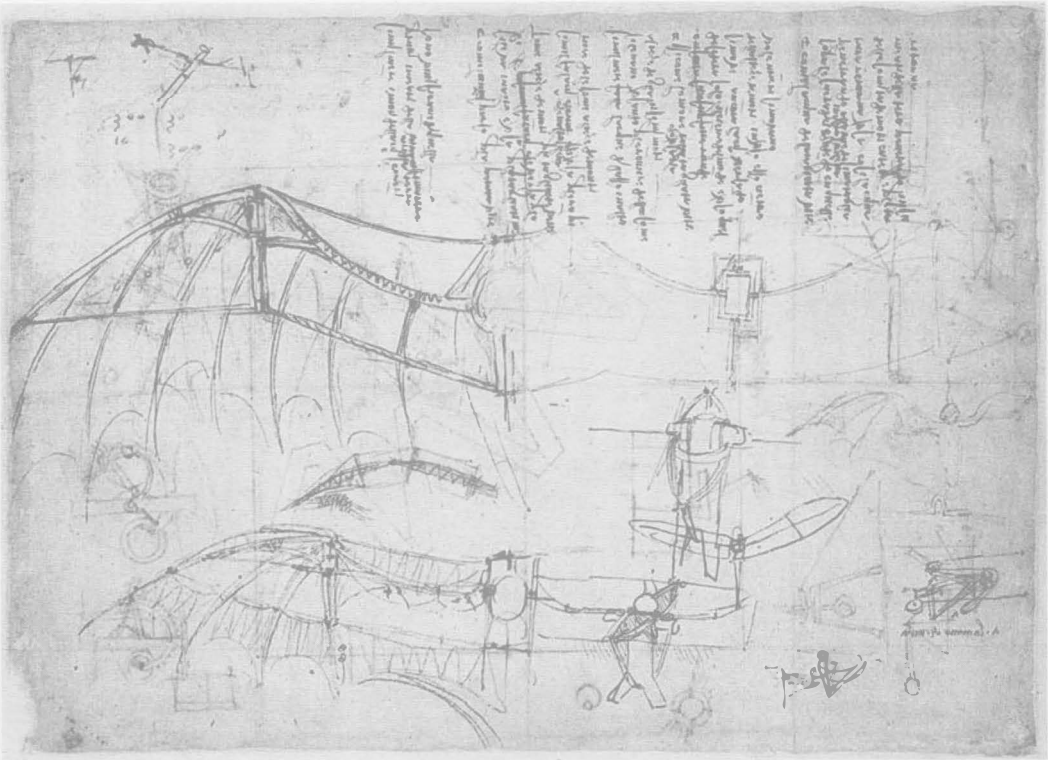
19. Bir Uçma Makinesi İçin Kanat Tasarımı , Milano, Biblioteca Ambrosiana, Codice atlantico, 858
