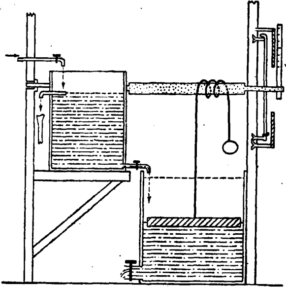
Şekil 9 - F.Maitzinger tarafından tasarlanmış büyük sarkaç denemesi
