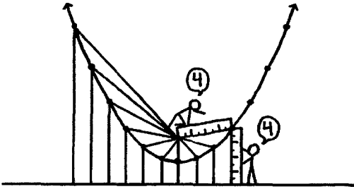
Şekil 1: Parabolün tanımı: bir noktaya ve bir doğruya eşit uzaklıktaki noktalardan oluşan eğri.
