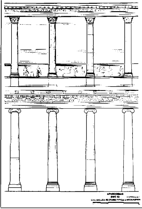
Resim 2. Aphrodisias, Sivil Bazilika, doğu sütun sırasının restore edilmiş görünüşü (P. Stinson, New York Üniversitesi Aphrodisias Kazıları).
