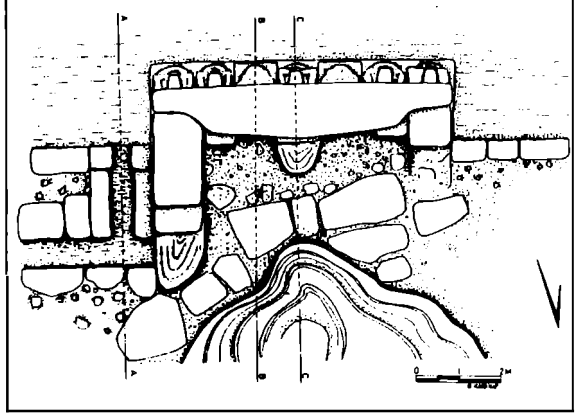
Resim 2b. Eflatunpınar Anıtı, üstten görünüm (Özenir 2000).
