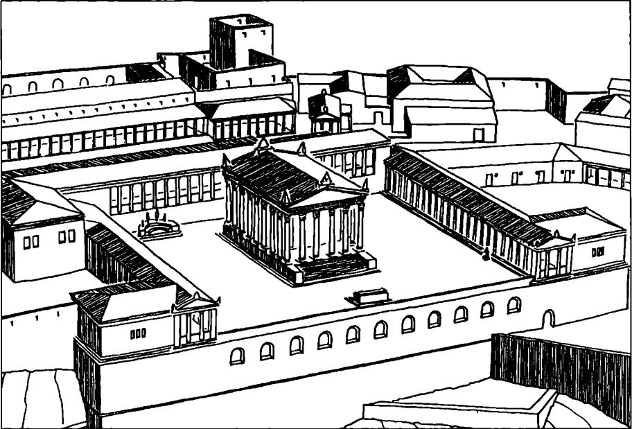
Resim 2. Bergama Traianus Tapınağı'nın rekonstrüksiyon çizimi (Radt 2002: 211).
