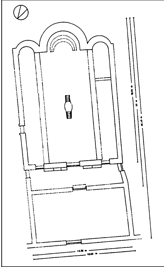
Resim 3. Akropol Bazilikası, rekonstrüksüyon planı (Ufuk Serin).
