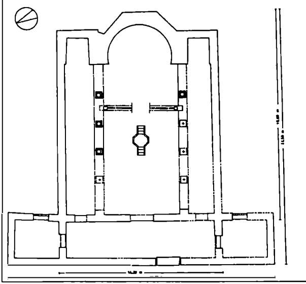
Resim 8. Agora Bazilikası, rekonstrüksüyon planı (Ufuk Serin).
