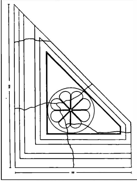
Resim 4. Akropol Bazilikası, ambona ait merdiven levhalarından biri, rekonstrüksiyon (Ufuk Serin).
