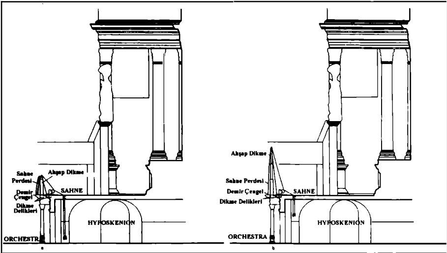
Resim 4. Perge tiyatrosu scaenae frons 'unun sahne perdesi için restitüsyon önerisi (Çizim ve Restitüsyon, Arzu Öztürk).
