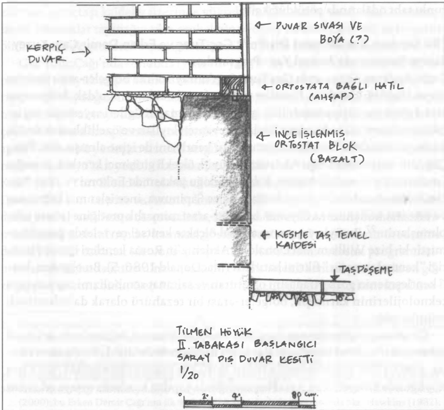
Resim 9. Tilmen Höyük, Orta Tunç Çağı sarayı kuzeybatı ortostatlarından sistem kesiti.
