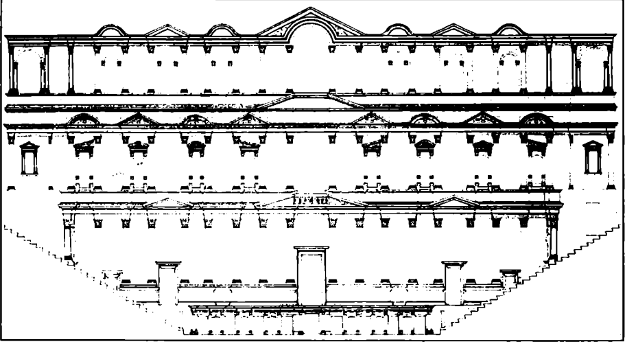
Resim 3. Perge tiyatrosu scaenae frons 'u için restitüsyon önerisi (Çizim ve Restitüsyon, Arzu Öztürk).
