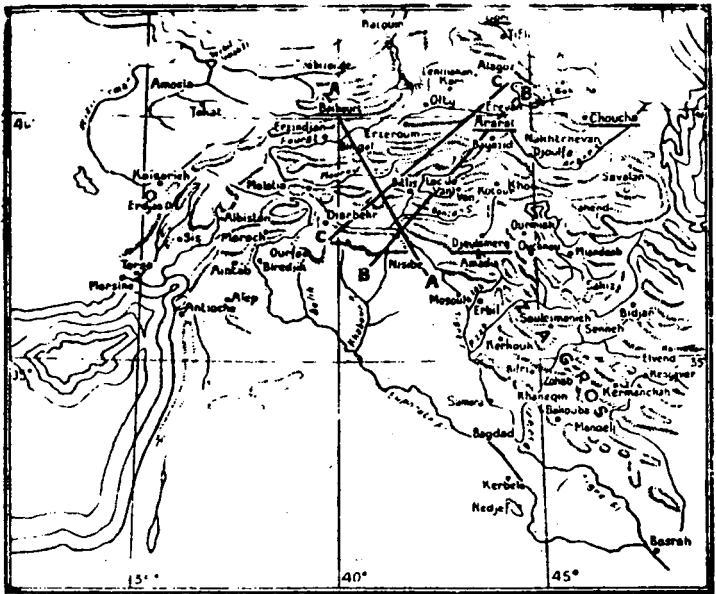
HARİTA 2. — Kürdistan'ın fiziki haritası. Gari, Bayburt, Şuşa ve Gulamerg isimlerinin altları, Anaratın merkezini gösterdiği bakla şeklindeki siralama çizilmiştir. A-A, B-B ve C-C profilleri için bak. Christoff'un haritası (4)
