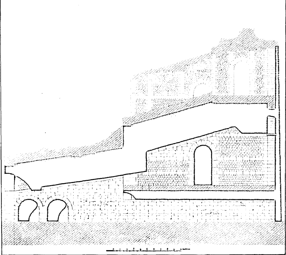
BERGAMA (PERGAME). AMFİTİYATRO'NUN BİR KISMININ CEPHE ÇİZİMİ VE KESİTİ
