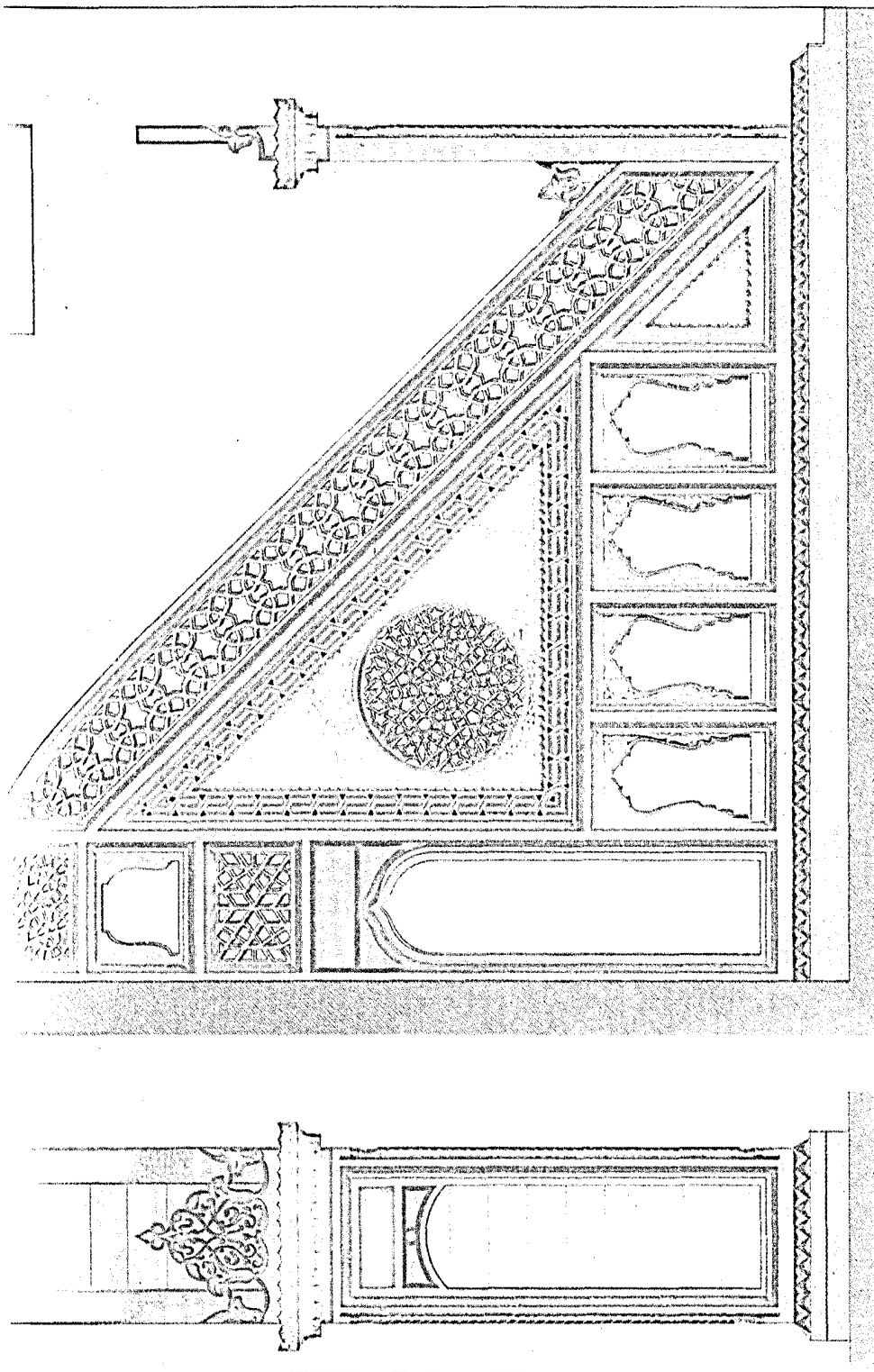
IZNIK (NICÉE). MINBER.
