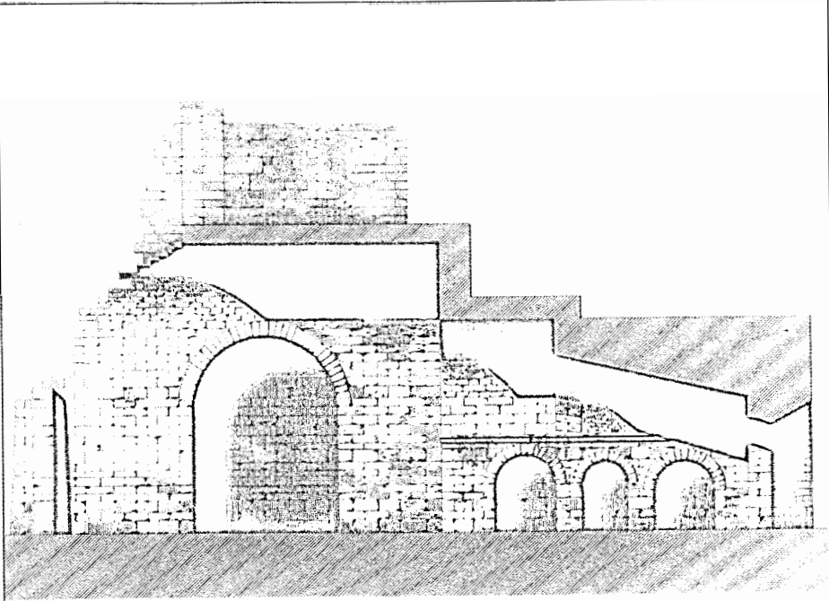
COUPE SUR LA GRANDE GALERIE DE L'AMPHITHÉÂTRE
