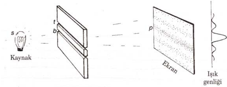
Tek renkli ışıqla yapılan çift yarık deneyi
