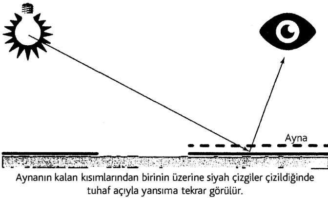
Şekil 4. Eksik yansıma
