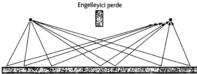
Şekil 3. Çok yollu yansıma
