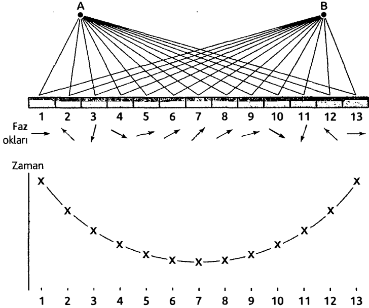
Şekil 5. Farklı yansıma yolları
