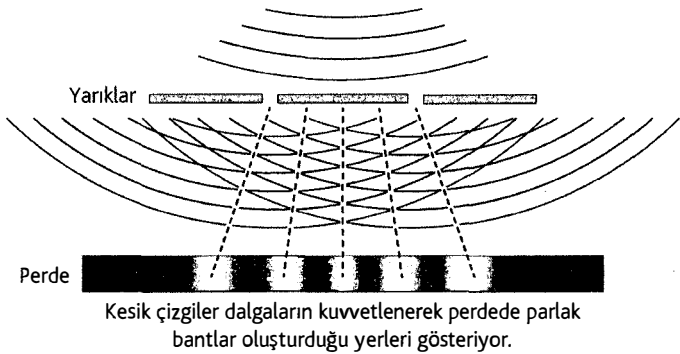
Şekil 1. Young yarıkları
