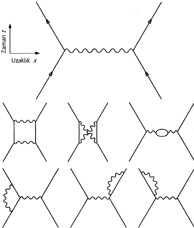
Şekil 6. İki basit elektron etkileşimini gösteren Feynman diyagramları
