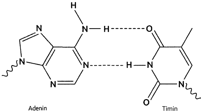
Şekil 2. Hidrojen bağı (kesik çizgiler) gösteren A-T baz çifti
