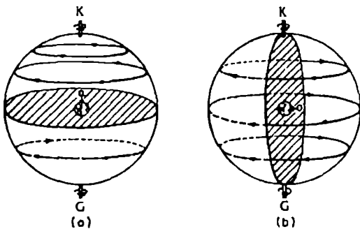
Şekil 12. İki küreli evrende (a) kuzey gezegen kutbundaki ve (b) ekvator'daki bir gözlemcinin gördüğü yıldız devinimleri.
