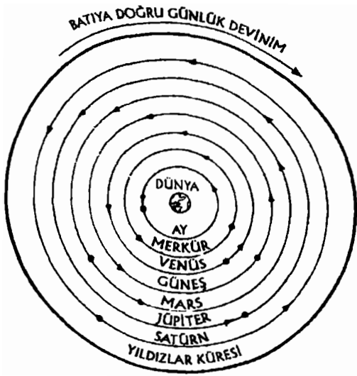
Şekil 16. İki küreli evrende yaklaşık gezegen yörüngeleri. En dıştaki çember, yıldızlar küresinin tutulum düzlemindeki kesitidir.
