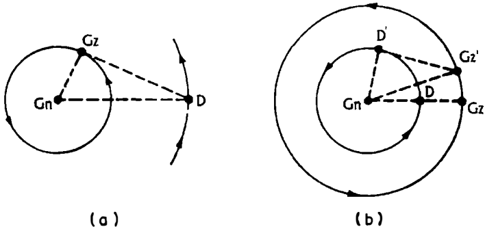
Şekil 36. Kopernikçi sistemde (a) bir alt gezegen için, (b) bir üst geze- gen için yörüngelerin görelî boyutlarının saptanması.
