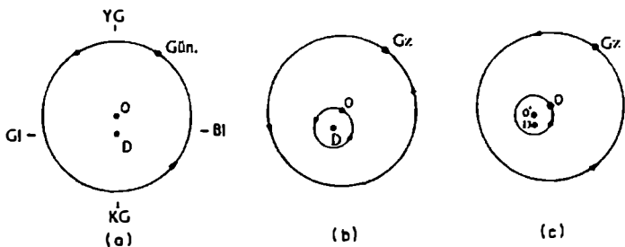
Şekil 24. Bir dış merkezli (eksantrik) (a), bir taşıyıcı çember üzerindeki bir dış merkezli (b) ve bir dış merkezli üzerindeki bir dış merkezli (c).
