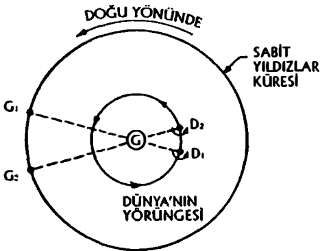
Şekil 28. Dünya Kopernikçi yörüngesinde D_1 'den D_2 'ye geldiğinde, merkezdeki Güneş'in, G , görünürdeki konumu yıldızlar küresine karşı G_1 'den G_2 'ye kayar.
