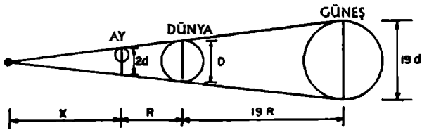
Şekil 59. Aristarkhos'un, bir Ay tutulması sırasında yapılan gözlemlere dayanarak, Ay'ın ve Güneş'in mutlak uzaklıklarını hesaplamak için kurduğu yapı.
