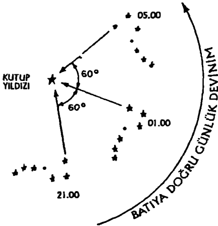
Şekil 5. Ekim ayının sonuna doğru bir gecede tavanın birbirini izleyen dört saatlik aralıklarla konumu.
