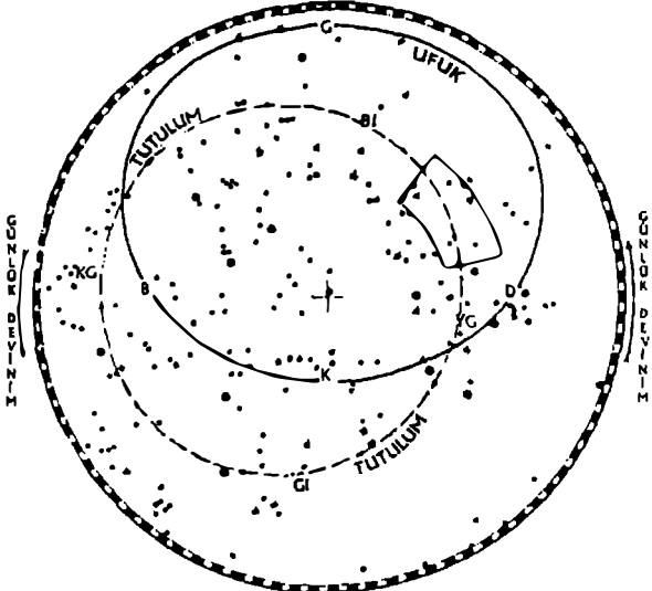
Şekil 8. Yaklaşık olarak 45° kuzey enlemindeki bir gözlemciye her zaman görünen büyük yıldızların tümünü içeren bir dolaykutupsal yıldız haritası. Haritanın geometrik merkezindeki arı işaret, gökkubunun yerini göstermektedir.
