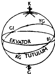
Şekil 13. Gökküre üzerinde ekvator ve tutulum.
