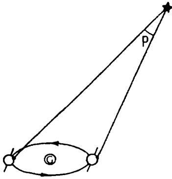
Şekil 30. Bir yıldızın yıllık paralaksı. Dünya yörüngesinde devinirken, yeryüzündeki bir gözlemci ile sabit bir yıldız arasındaki doğru tam olarak kendisine paralel kalamadığı için bu yıldızın yıldızlar küresindeki görünüşteki konumu altı aylık bir zaman aralığında bir p açısı kadar kayacaktır.
