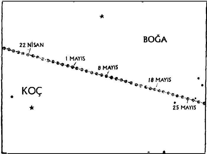
Şekil 9: Güneş'in Koç ve Boğa takımyıldızları arasındaki devinimi. Daireler Güneş'in Nisan ortasından Mayıs sonuna dek birbirini izleyen akşamlarda günbatımında yıldızlar arasındaki konumunu belirtmektedir.
