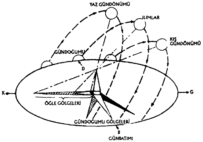
Şekil 2. Gündoğumu konumu, Güneş'in öğle yüksekliği ve gnomonun gölgesinin mevsimlik değişimi arasındaki bağıntı.
