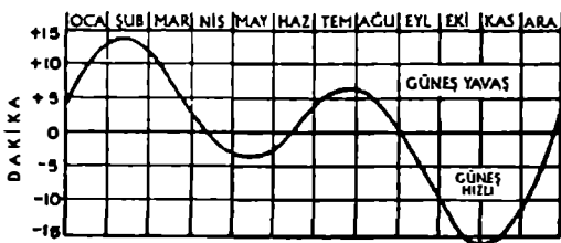
Şekil 53. Ortalama ve görünen Güneş zamanları arasındaki farkın yıllık değişimini gösteren bir zaman denklemi grafiği.
