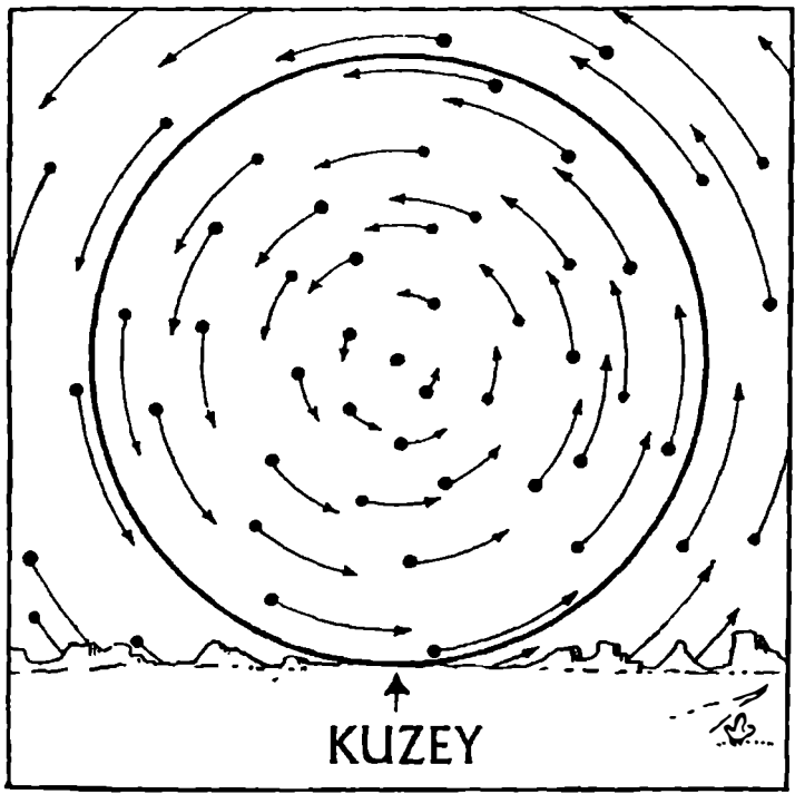
Şekil 6. Kuzey göğünde iki saatlik bir sürede belli yıldızların çizdiği bir grup kısa dairesel yay. Ufka teğet olan koyu çember, dolaykutupsal yıldızları, doğup batan yıldızlardan ayırır.
