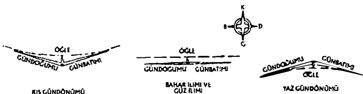
Şekil 3. Kuzey sıcak kuşakta gnomomun gölgesinin değişik mevsimlerdeki günlük devinimi.
