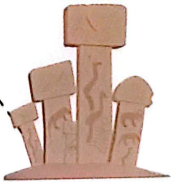
Göbeklitepe (Şanlıurfa)
