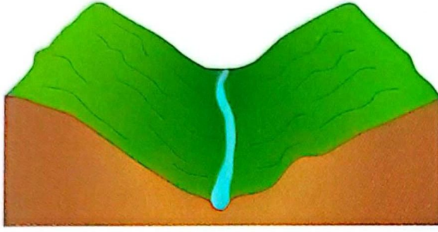
← Çentik Vadi
