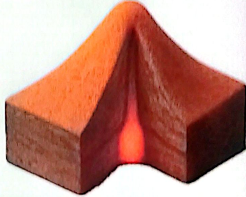
Kül Konisi!
