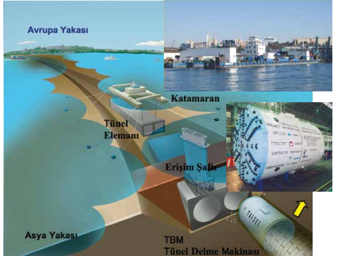
BATIRMA TÜP GÜZERGAHINDA HENDEK KAZISI.
