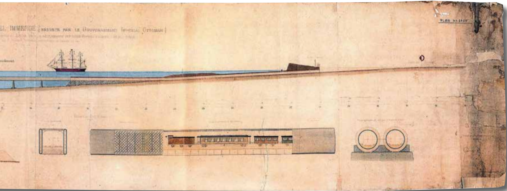
SARAYBURNU-ÜSKÜDAR ARASINI TÜP GEÇİTLE BAĞLAMASI PLANLANAN VE FRANSIYALI DEMİRYOLU MÜHENDİSLERİNDEN S. PREAULT TARAFINDAN SULTAN ABDÜLHAMİT'E SUNULAN "DENİZ ALTI ÇELİK TÜNELİ" PROJESİ (TAKSİM BELEDİYE KÜTÜPHANESİ ARŞİVİ).
