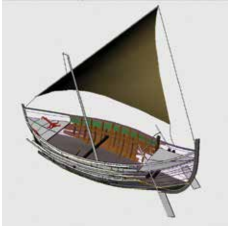
YK 1 BATIĞININ ÜÇGEN LATİN YELKEN VE DÜMEN KÜREKLERİ İLE BİRLİKTE ÜÇ BOYUTLU ÖN REKONSTRÜKSİYONU.
