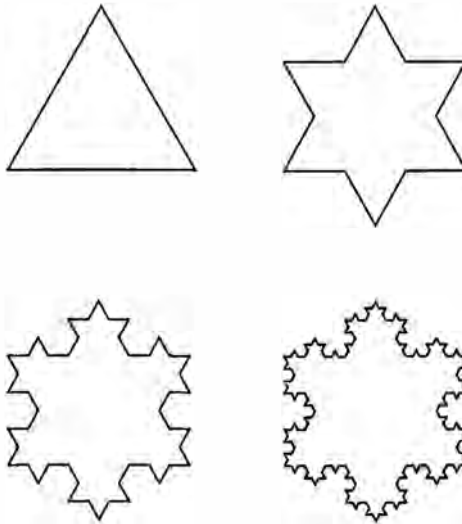
RESİM 7: Koch’un kar tanesi. Eşkenar bir üçgenle başladıktan sonra sürekli olarak her kenarın ortasından üçte birinin çıkartılarak, yerine çıkartılan parçadan iki tane eklenmesi yoluyla oluşturulan basit bir fraktal biçimdir. En çarpıcı özelliklerinden biri, kenar uzunluğu sonsuz iken alanının sınırlı olmasıdır.
