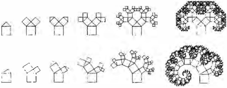
RESİM 6: Fraktal şekillerin en bilinenlerinden “Pisagor ağacı”.
