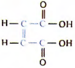
Maleik asit
