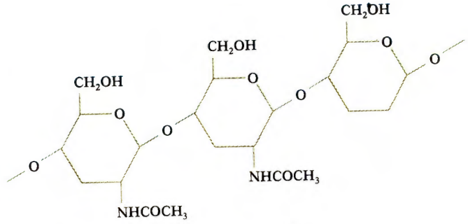
Kitin
