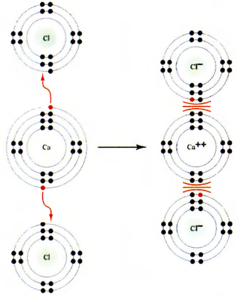
2.12 Kalsiyum ve klor arasında iyonik bağ
