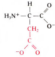
Serin (Ser)
