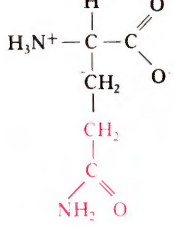
Glutamin (Gln)
