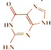
Guanin
