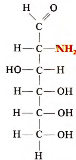
Glukozamin
