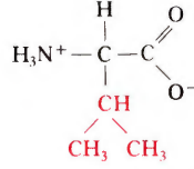
Valin (Val)
