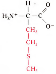
Metionin (Met)
