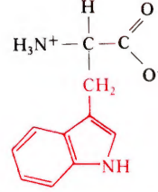
Triptopan (Trp)
