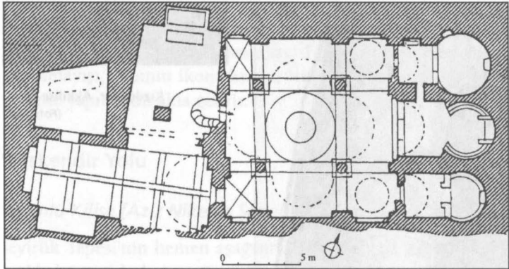
ÇİZİM 16 Akkilise planı. (Thierry: 1994)
