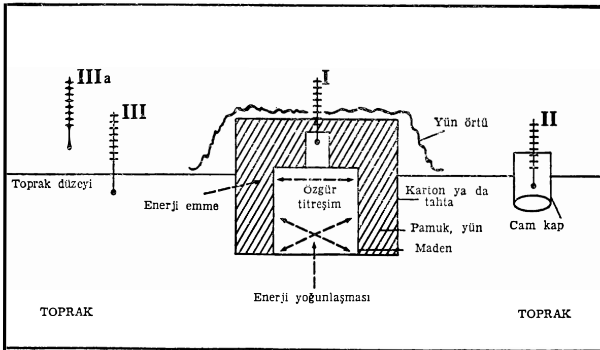
Şekil 12. — To-T ısı ayrımının açıkavada ölçülmesi deneyi (bu deney 16-17 Şubat 1941'de gerçekleştirilmiştir).
