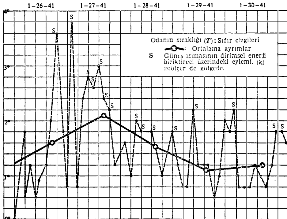
Şekil 13. — Penceresi açık bir odada ısı ayrımlarının ölçülmesi.
