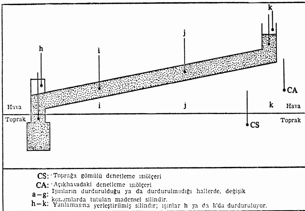
Şekil 14. — T_o - T ayırımını toprakta ve havada ölçmenin değişik yöntemleri.
