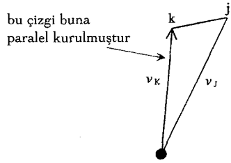
(hız diyagramı)
