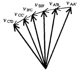
(hız diyagramı)
