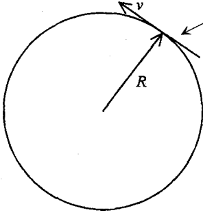
(dairesel yörünge)
