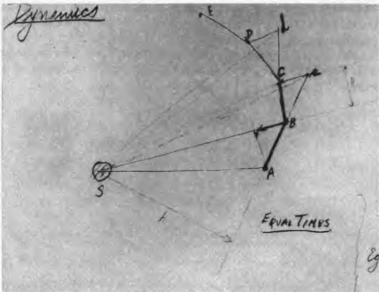
Feynman'ın diyagramı
