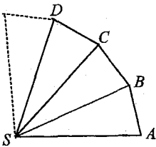
(yörünge diyagramı)
