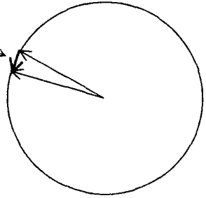
(hız diyagramı)
