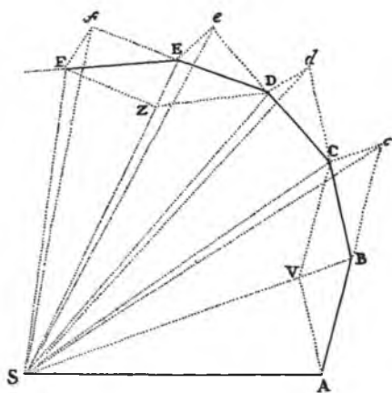
Newton'un diyagramı
