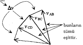
(hız diyagramı)
