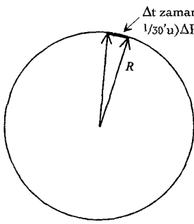
(yörünge diyagramı)
