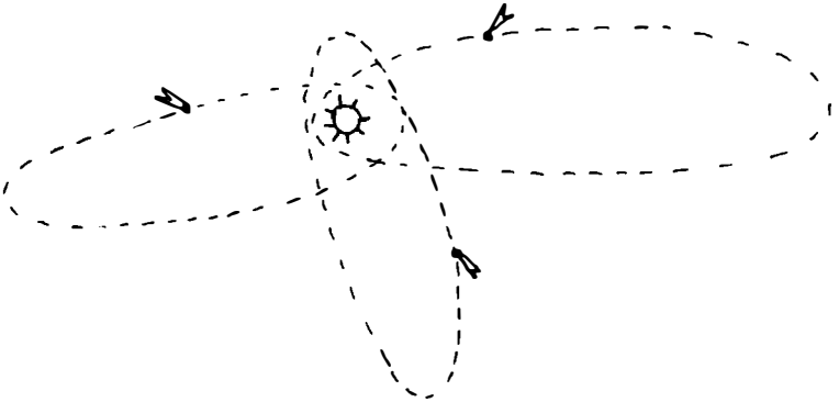
Kuyruklu yıldızlar: Messier'nin başlıca takıntısı.
