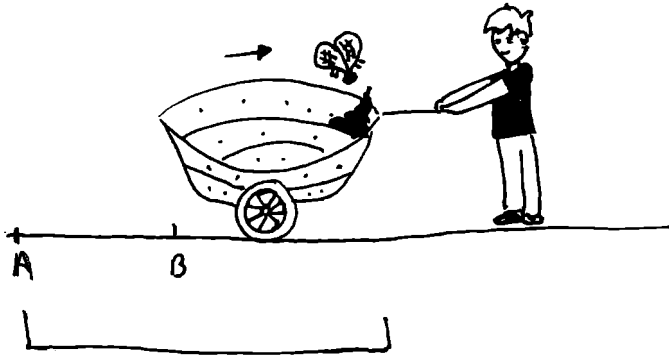
Sineğin katettiği mesafe
