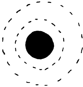
Rutherford'un atomu
