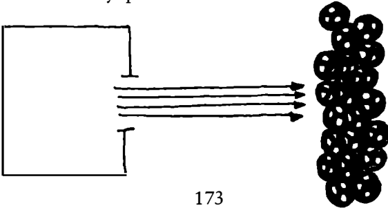
Thomson'ın atomlarıyla deney
