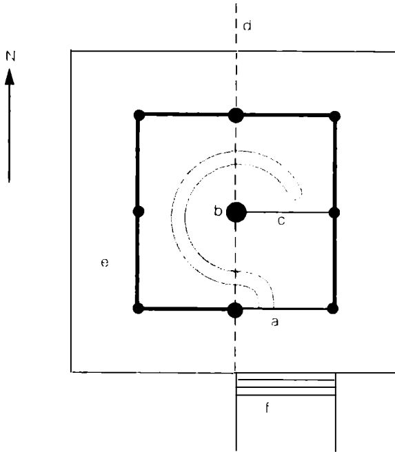
Resim 10 / Büyük İzuma Tapınağının tanrılar holünün temel planı. a) Giriş, b) Çatıya kadar yükselen orta sütun, "saygın yürek sütunu", c) Ayırıcı duvar, arkasında tanrılar makamı, d) Çatı hizası, e) Çerçeve dolaşan veranda, f) Merdivenli giriş, 15 basamaklı. (Büyük İzuma Tapınağının mimarisi için ayrıca bkz. 1988, 120 ve devamı.)
