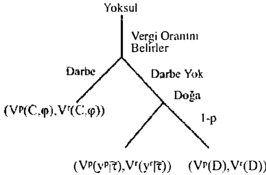
Şekil 7.1. Darbe Oyunu
