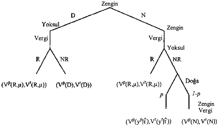
Şekil 6.1. Demokratikleşme Oyunu.
