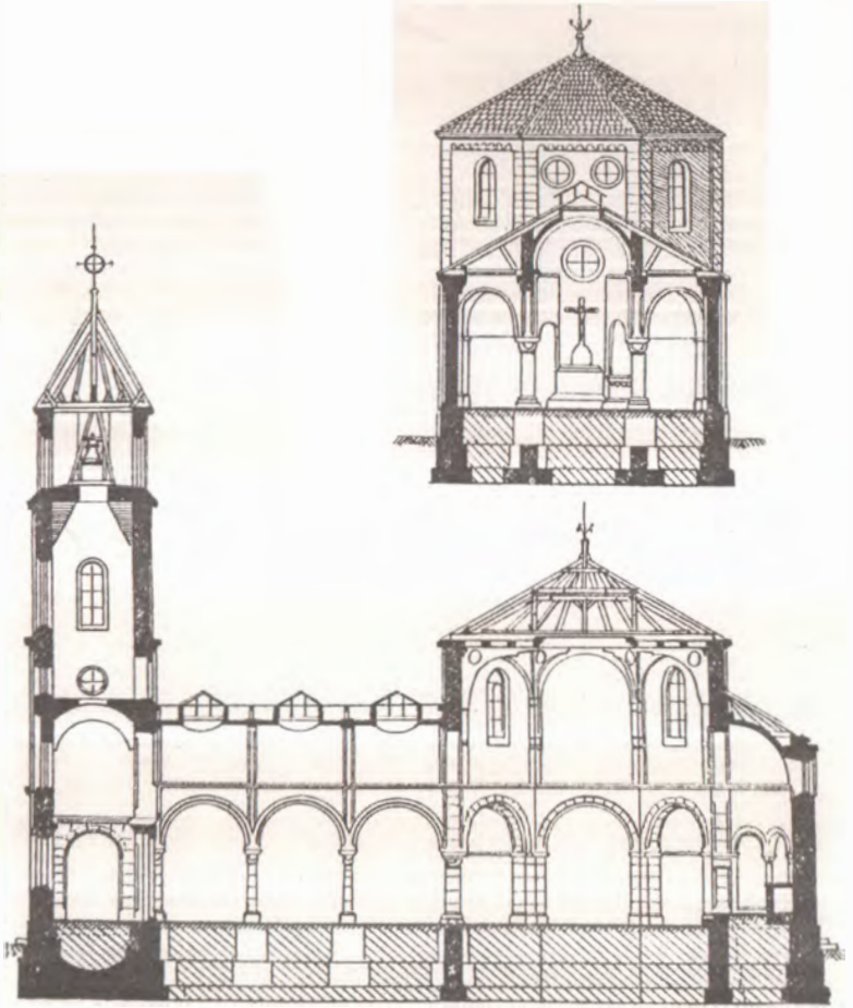
İzmir Alman Kilisesi'nin yandan ve önden mimari kesitleri.
