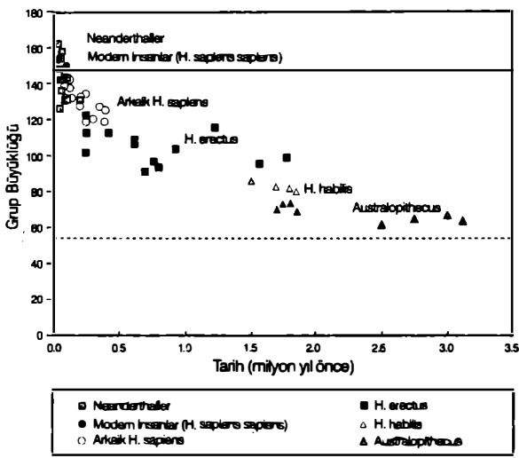
Şekil 4. Grup Büyüklüğü, Beyin Büyüklüğü ve Evrim Tarihi Arasındaki İlişki
