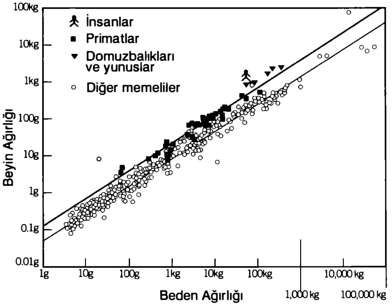
Şekil 27. Karşılaştırmalı Beyin Büyüklüğü
