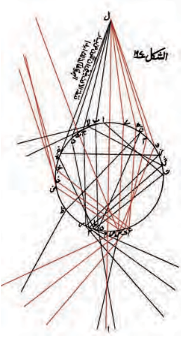
Kemâleddin el-Fârîsî, Tenkih , Haydarabad, Cilt 2, Resim 192.
