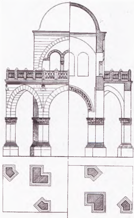
76. Hırbetü'l-Mefcer. Ön avludaki havu- zun rekonstitüsü (Robert Hamilton, Khirbat al Mafjar 'dan alınma).
