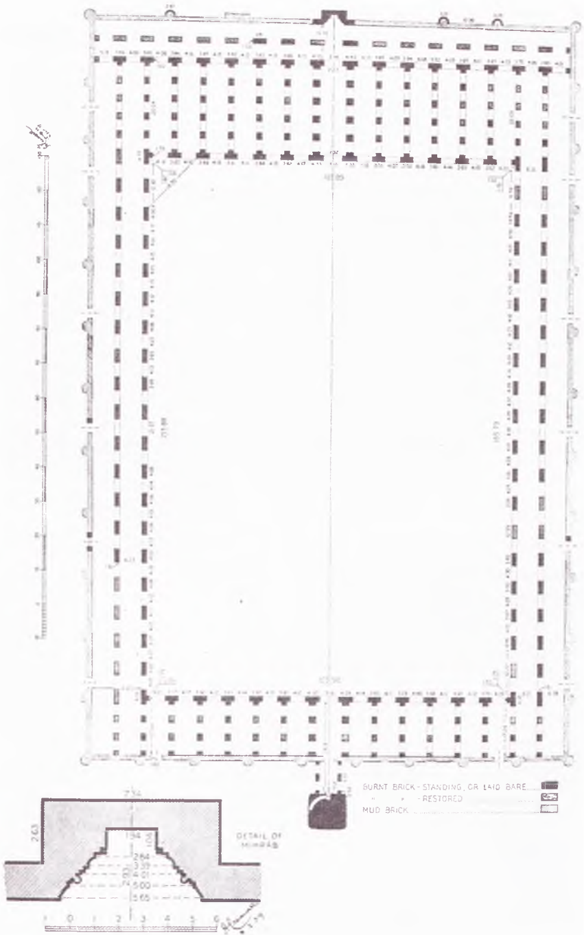
36. Samarra. Ebu Dulaf diye bilinen cami, 9. yüzyıl ortaları, plan (K. Archibald C. Creswell, Early Muslim Architecture , cilt
