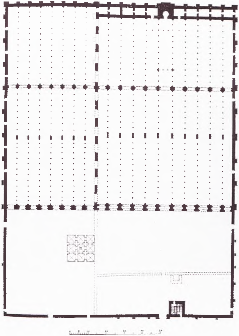
27. Kurtuba. Cami, gelişme şeması ( Ars Hispaniae , cilt III'den alınma).
