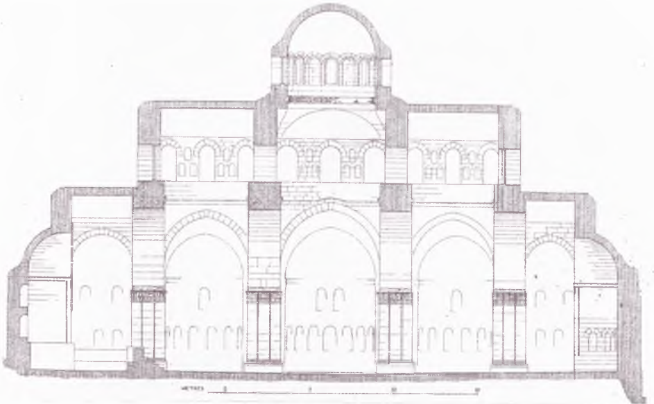
72. Hirbetü'l-Mefcer. Hamamın rekonstitüsyonu (Robert Hamilton, Khirbat al-Mafjar 'dan alınma).
