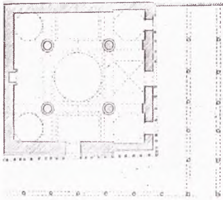
50. Hezare Cami, 10. yüzyıl, plan.
