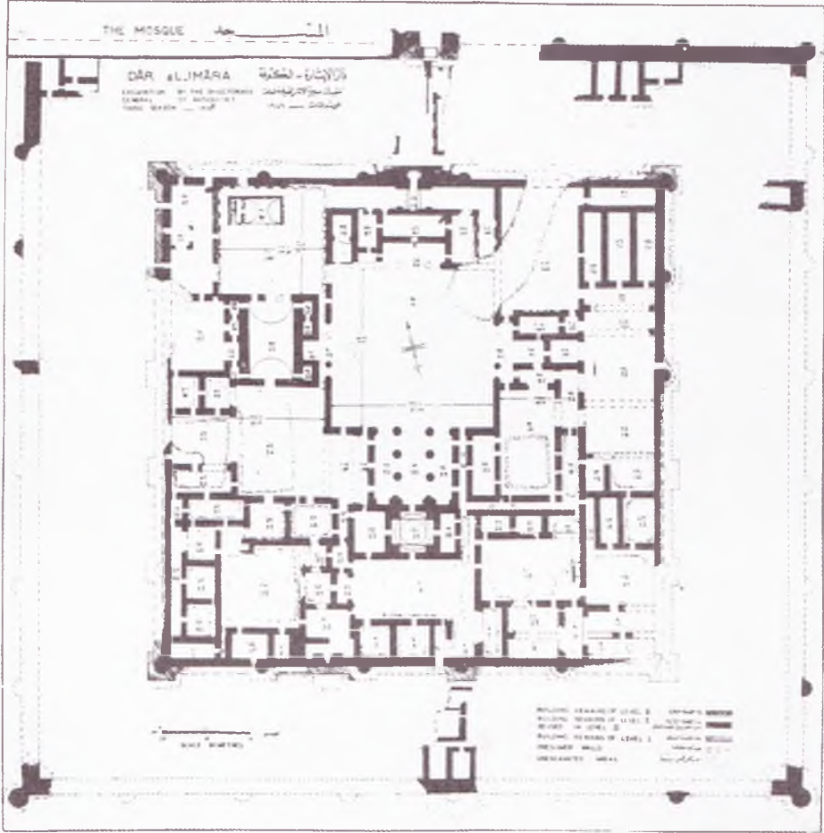
64. Kûfe. Saray, 7. yüzyıl sonu-8. yüzyıl başı, plan (Muhammed Ali, Sumer 12 'den alınma).
