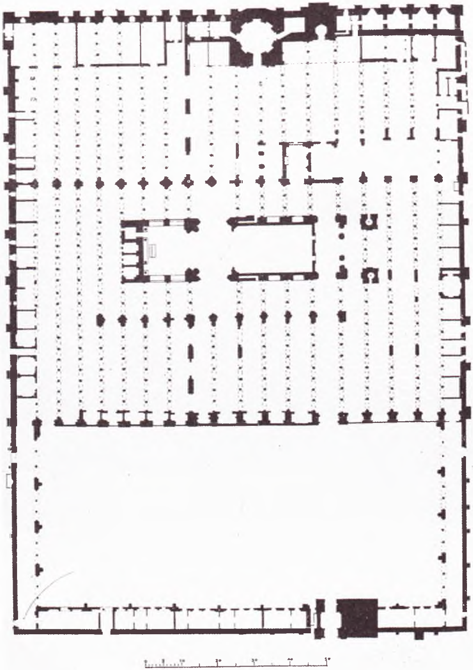
26. Kurtuba. Cami, 8.-10. yüzyıllar, plan ( Ars Hispaniae , cilt III'den alınma).
