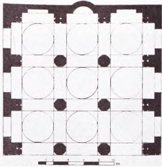
39. Belh. Cami, 9. yüzyıl, plan (Lisa Golombek, Oriental Art 'tan alınma).
