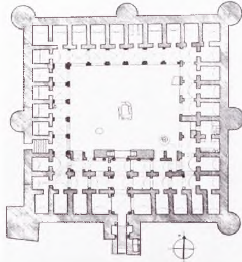
51. Susa Ribat, 8. yüzyılın ikinci yarısı, zemin kat planı (Lézine, Le ribat de Sousse 'dan alınma)
