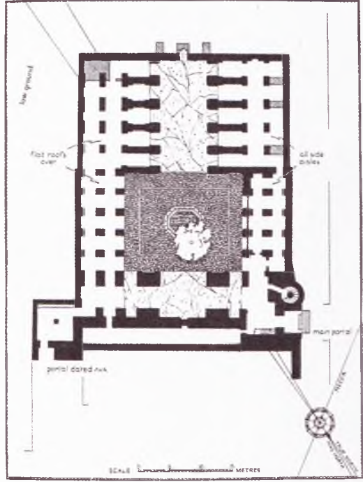
49. Niriz Cami, 10. yüzyıl, plan (Arthur U. Pope ve Phyllis Ackerman [yay. haz.], A Survey of Persian Art , cilt II'den alınma).
