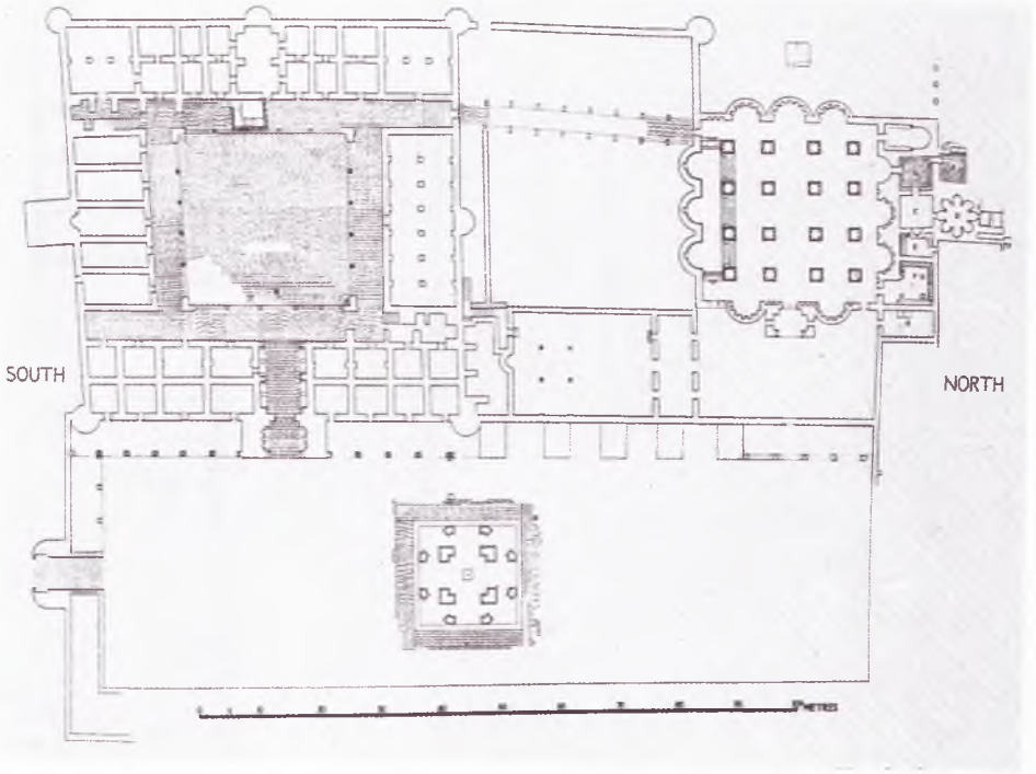
60. Hırbetü'l-Mefcer. Saray, cami ve hamam, 8. yüzyılın ilk yarısı (Robert Hamilton, Khirbat al- Mafjar 'ından alınma).
