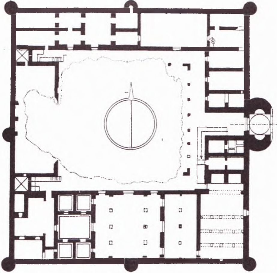
58. Hırbet Minye. Saray, 8. yüzyıl başı, plan (Oswin Puttrich-Reignard'dan alınma).
