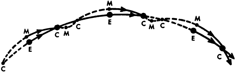
Çizim 48. Dünyayla ayın yörüngelerinin çekimsel üst üste binmesi. Ay (M), yerkürenün (E) merkezine (C) doğru düşmektedir.
