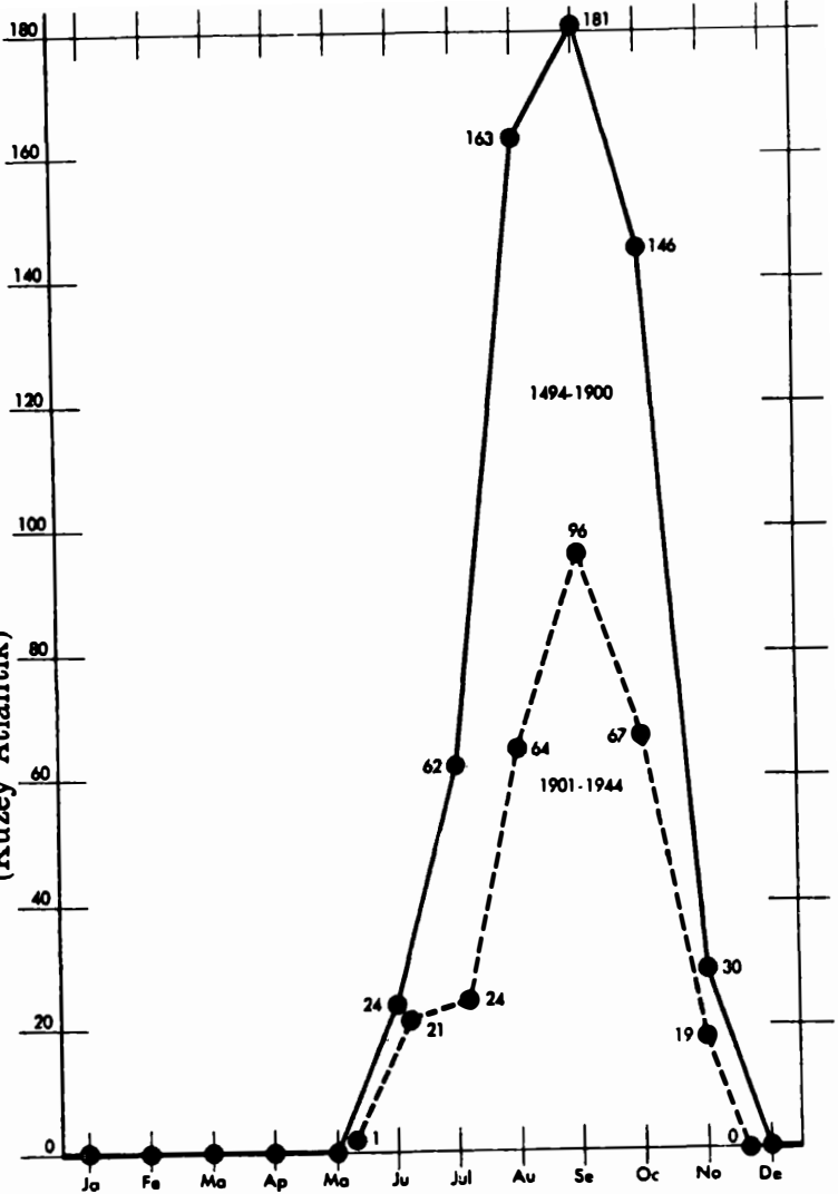
Çizim 47 Ocakla Aralık arasında dönence kasırgalarının sıklığını gösteren eğri
