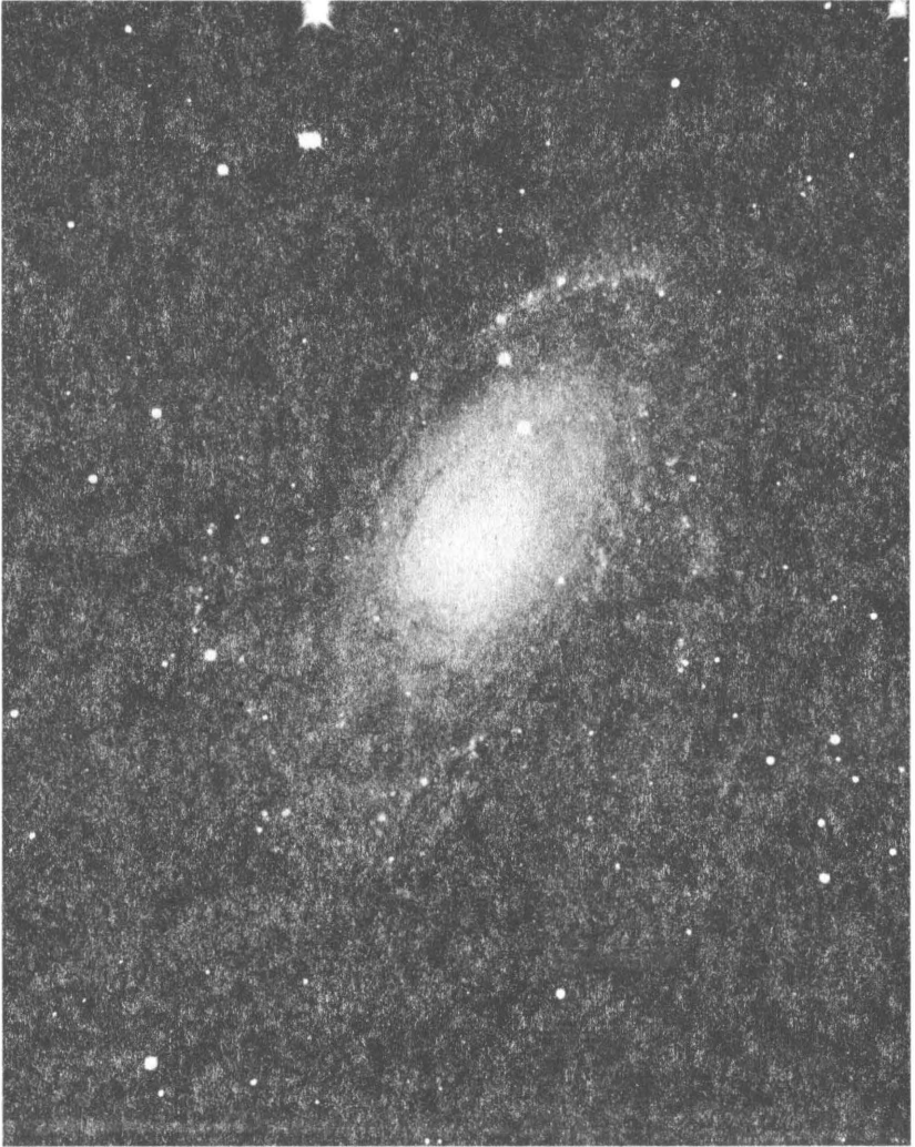
Çizim 35. Messier 81, G 10 sarmalı (foto: Mount Wilson)
