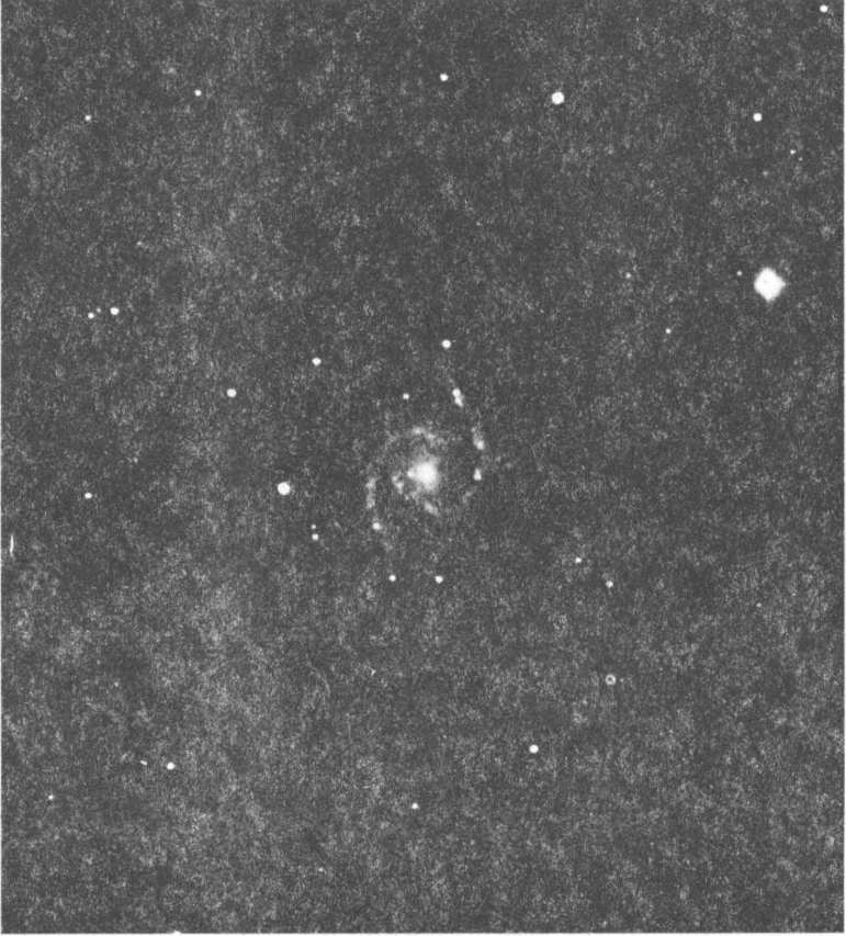
Çizim 33. Harvard'da aynalı bir teleskop yardımıyla saptanmış kuzey yarımküredeki NGC 1566 sarmalı
