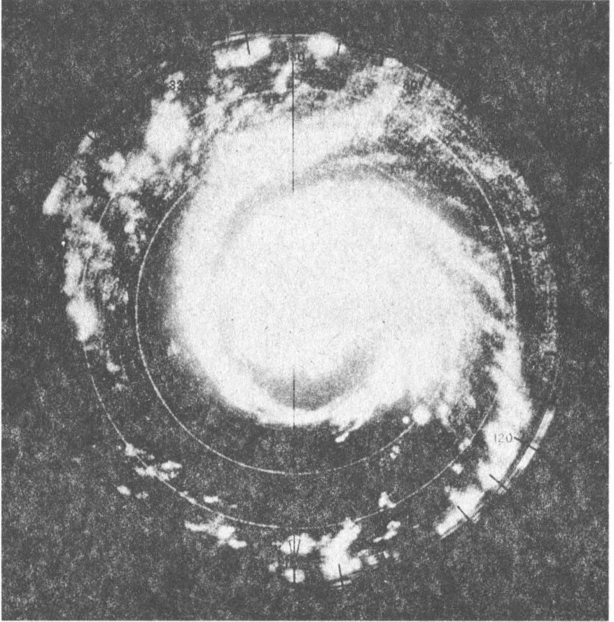
Çizim 41. 21 Eylül 1948 Kasırgası, saat: 1131 (U. S. Naval fotoğrafı, Nr. 706.634)
