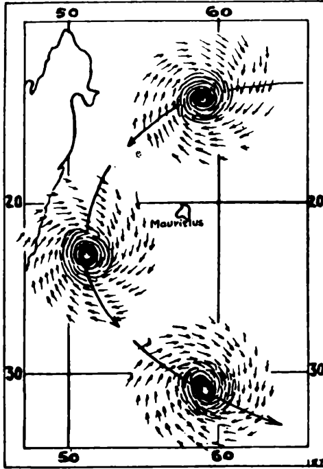
Çizim 45. Güney yarıkürede dönence bölgesindeki bir kasırgada rüzgârların yönü ve yolu (Tannehill, Hurricanes, s. 6)
