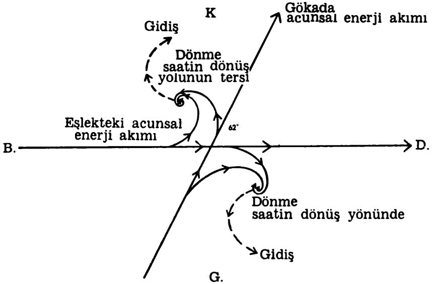
Çizim 43. Kasırgaları oluşturan güçler ve izledikleri yol
