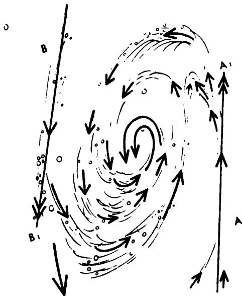
Çizim 36.35 numaralı fotoğraftan çıkarılmış, iki dirimsel enerji akımının yönünü ortaya vuran yalın çizim
