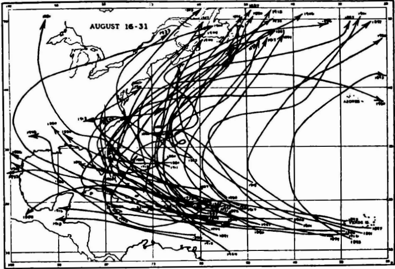
Çizim 46. 16-31 Ağustos 1874-1933 arasında, yüksek güçte dönence kasırgalarını gösteren çizim
