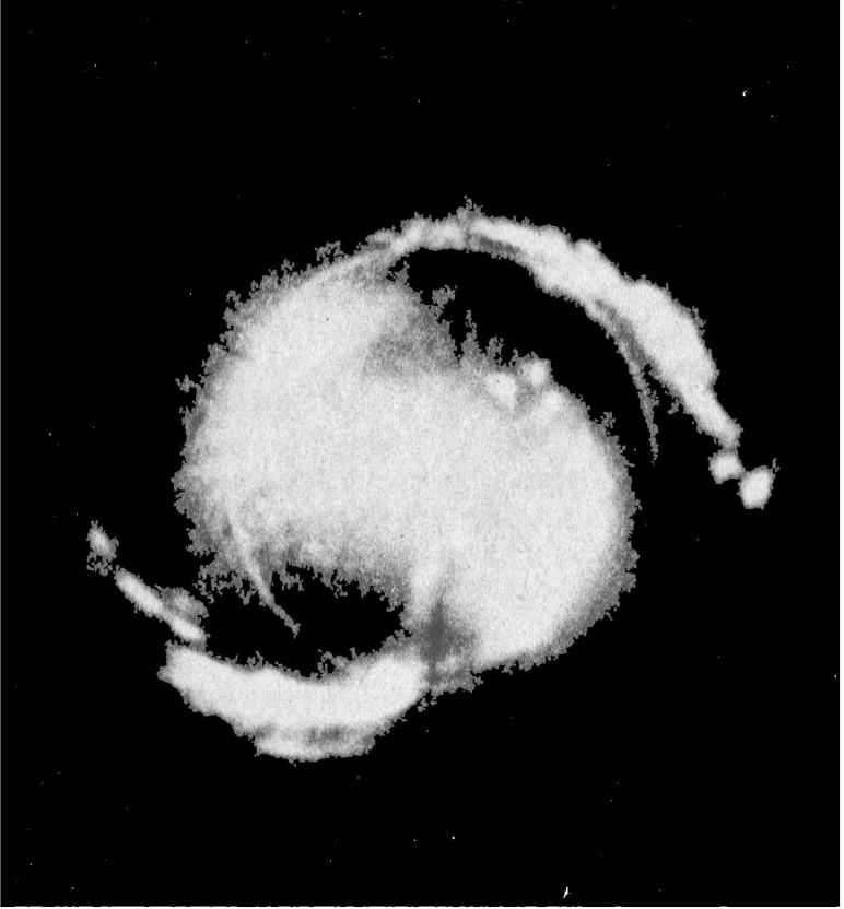
Çizim 40. 22 Ağustos 1949 Kasırgası
