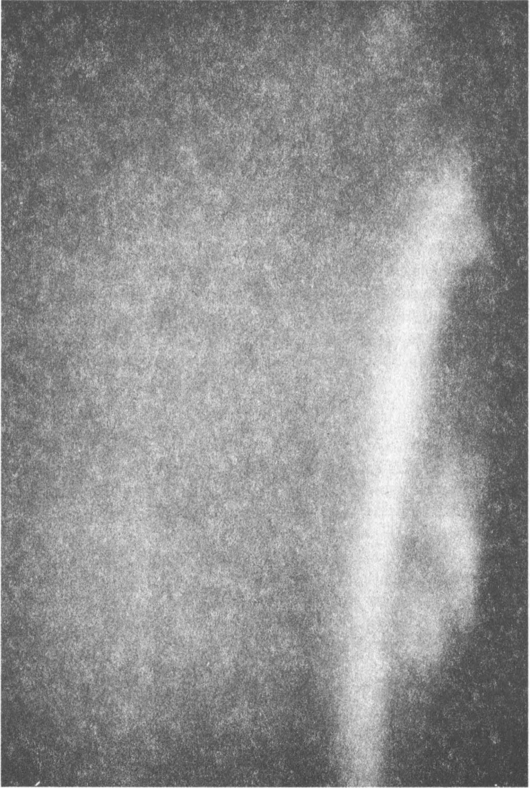
Çizim 37. Maine ilinin Rangeley ilçesindeki Orgonon'da 5 Eylül 1950'de gözlenen kutup ışığı
