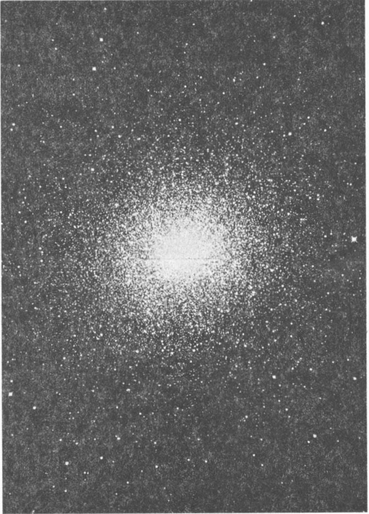
Çizim 29. Messier 13, "Büyük Herkül Kümesi" (foto: Mount Wilson)
