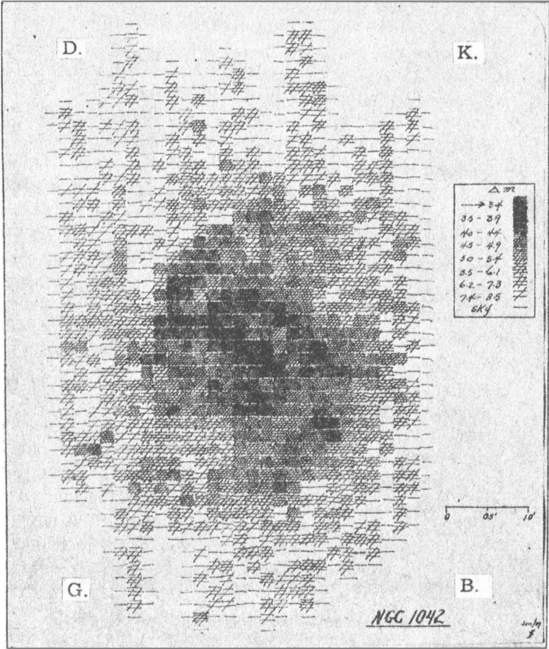
Çizim 32. Bayan F. S. Patterson tarafından, Shapley'in "Galaxies" (Gökadalar'daki) uyarılarına göre Oak Ridge'de çekilmiş bir resme dayanarak sarmal biçimli bir kasırganın "Microdensitor" çözülmesi
