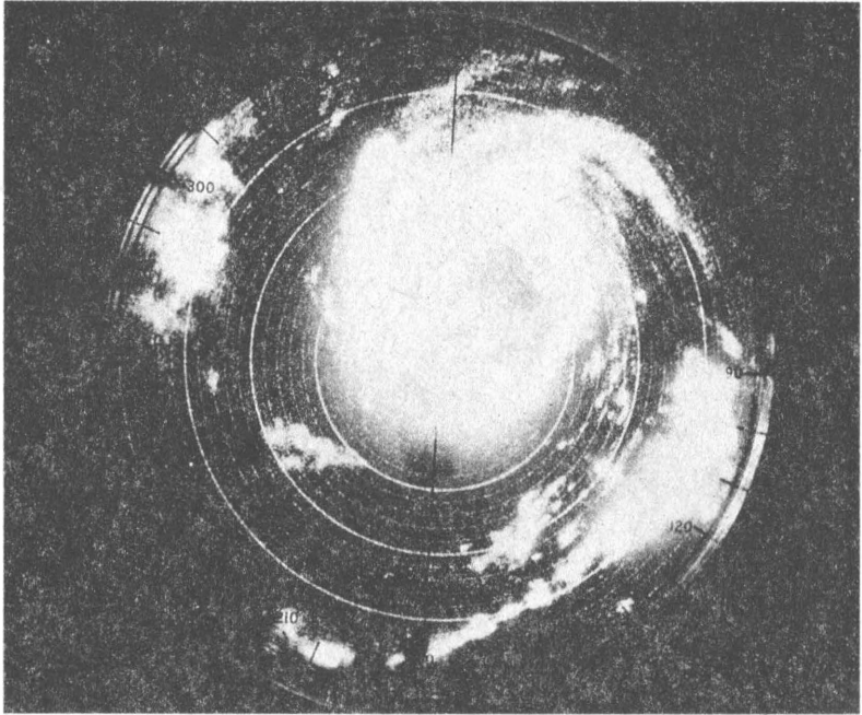
Çizim 42. 21 Eylül 1948 Kasırgası, saat 13 (U.S. Naval fotoğrafı, Nr. 706.635)
