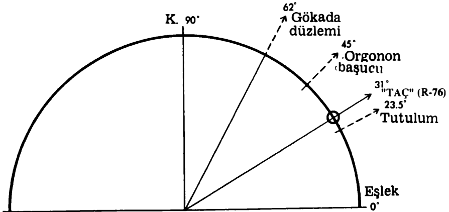
Çizim 39. "Taç" (R-76) ile gökada ve eşlek düzlemi arasındaki açıları gösteren çizim.
