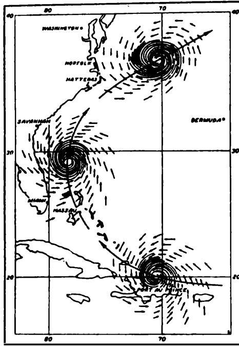
Çizim 44. Kuzey yarıkürede dönence bölgesindeki bir kasırgadaki rüzgârların yönü ve yolu (Tannehill, Hurricanes, s. 5)
