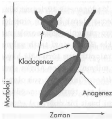
Şekil 7. İki tip türleşme modeli. Anagenetik türleşmede bir tür zaman sürecinde birikimli olarak değişerek başka bir türe dönüşür; dolayısıyla tür sayısı artmaz ve ata tür ortadan kalkar. Kladogenetik türleşmede ise ana gruptan ayrılan alt popülasyon izole olarak farklı bir türe dallanarak dönüşür; ana tür yok olmayabilir ve tür sayısı artar.
