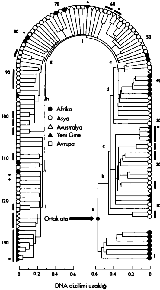
Şekil 8. Rebeca Cann ve ekibinin 147 modern insana ait mtDNA'larda 33 farklı varyasyonu tespit ederek oluşturdukları evrim ağacı modeli. mtDNA içindeki en belirgin çeşitlilik Afrikalı grup içinde görülür.
