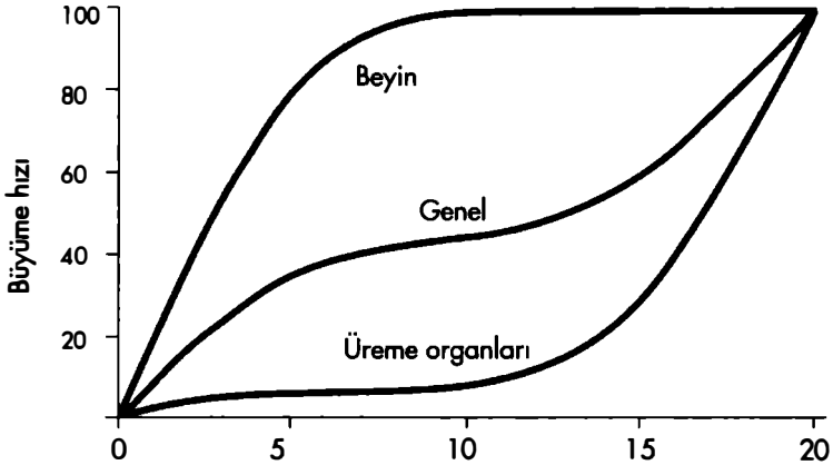
Şekil 27. Beyin, genel vücut yapısı ve üreme organları ağırlığında yaşla gözlenen allometrik büyüme
