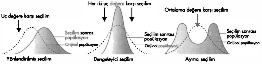
Şekil 5. Bir popülasyon üzerinde etkili olan üç tip doğal seçim mekanizması
