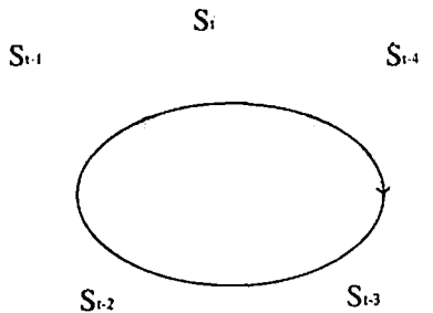
Şekil 1.2 Kapalı zaman modeli
