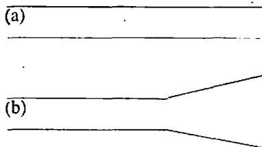
Şekil 7.1 Belirlenimli ve belirlenimsiz evrenler
