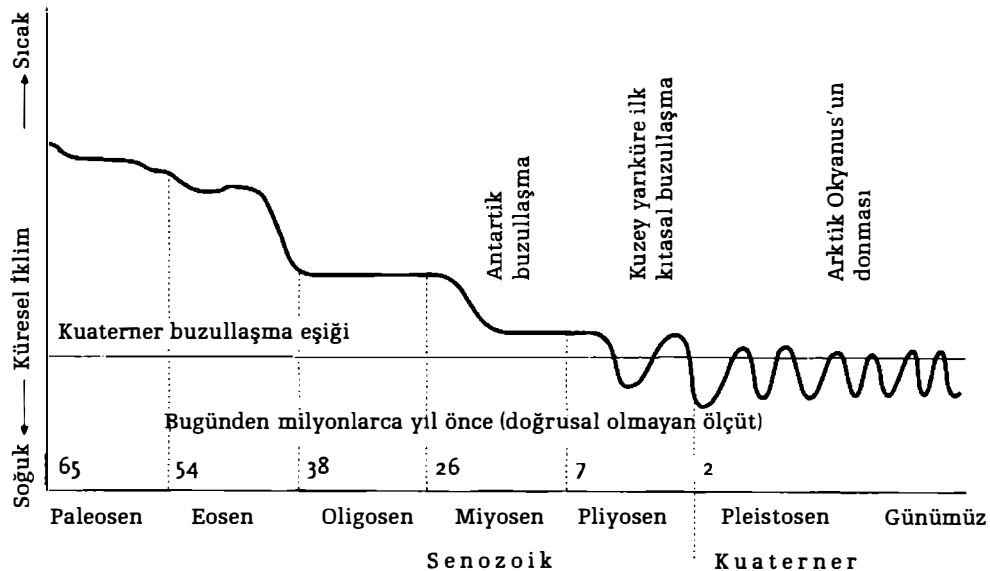
Şekil 8.1: 65 milyon yıl öncesinden, Paleosen dönemden bu yana küresel sıcaklığın düşüş eğrisi. Yatay zaman aralıklarının çizgisel olmadığına dikkat ediniz. Bu nedenle daha yakın dönemdeki varyasyonlar, ki büyük oranda Milankoviç sürecinin sonuçlarıdır, daha net görünmektedir. (J. Andrews, B. S. John (ed.), Winters of the World , David & Charles: Newton Abbot, 1979, yalnızca şema değiştirilerek alıntılanmıştır.)
