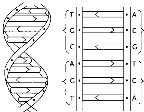
Şekil 2.1: Genetik kod çift sarmal oluşturmak için bir araya gelen DNA parçası boyunca yazılmıştır. Bazılar birbirlerini tamamlayan çiftler halinde oldukları için, her bir sarmal kendi eşini üretebilir.
