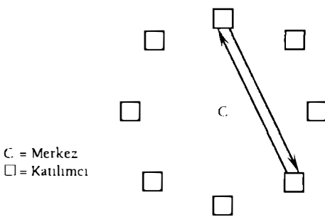
Şekil 8.2.2 Sohbet kalıbı
