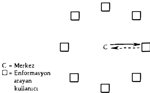
Şekil 8.2.3 Danışma kalıbı
