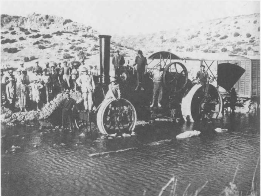
Kabara'nın Drenajı 1922-26: (i) Operasyon öncesi inceleme (ii) Pompa motoru ve çalışma ekibi
