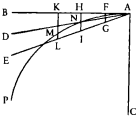
Şekil 11- AB teğeti, başlangıcındaki A noktasında Yerküre'yle çok dar açı oluşturması nedeniyle cisimlerin savrulup gitmesini zorlaştırmaktadır. AB çizgisi üzerindeki AF, AH, AK, belirli süreleri ifade ediyor; FG, HI, KL, sözünü ettiğimiz sürelerde cismin, ivme dolayısıyla, kazandığı hızı anlatıyor. Yerküre kavisini temsil eden AP çizgisini çekince bu çizginin FG, HI, KL sonlarına ulaşmadan önce kaviste M, N, O noktalarında
