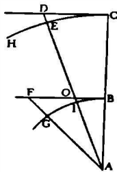
Şekil 14- Galileo aynı hızla dönen, biri küçük iki tekerin teğetlerini kıyaslıyor ve küçük tekerdeki bir cismin savrulup kaçmaması için aşağı çekme gücünün daha büyük olması gerektiğini kanıtıyor. Böylece, tekerin çapı büyüdükçe ve son tahlilde, Yerküre çapı da olunca, yeryüzündeki cisimlerin Yerküre'nin dönme hareketi nedeniyle savrulup gitmesinin imkânsızlığını kanıtıyor.
