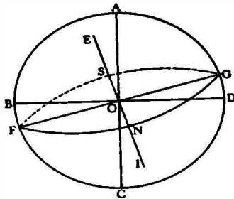
Şekil 23- Güneş'e ait bir önceki şekilde lekelerin 6 ay süreyle geçirdikleri değişiklik anlatılmıştı. Şimdi de diğer 6 ayda, yani Yerküre'nin ekseninin 23,5 derece eğik oluşu nedeniyle Güneş'in bizlere değişik açıdan görünüşü anlatılıyor.
