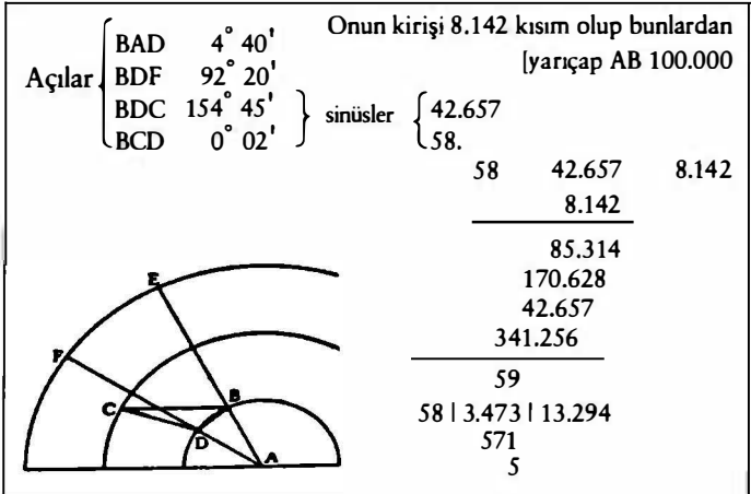
Şekil 18- Tanınmış birkaç astronomin paralaks bulguları. A Yerküre merkezi, B Langravio'nun rasat yaptığı yer, D Tycho'nun gözlem yeri. C yeni yıldızın yeri, BCD açısı paralaks farkı.
