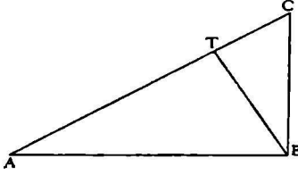
Şekil 5- Anlatılması çok güç olanı Galileo kolayca anlatır. “Eylemsizlik Kuramı”nı eğik düzlem sayesinde bulmuştur. Düşeydeki B’ye yakın bir noktadan harekete başlayan bir cismin, A’ya uzak noktadan harekete başlayan bir cisimden, Eylemsizlik Kuramı nedeniyle daha geç varması mümkündür.
