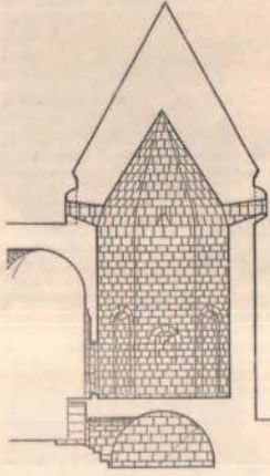
Kümbet kriptası yan kesiti
