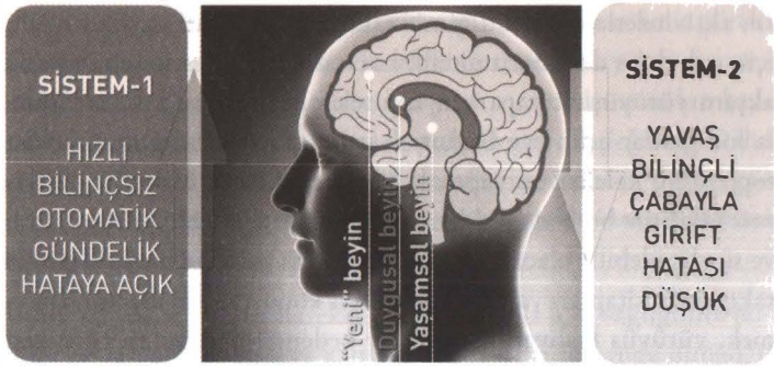
GÖRSEL 10: Beynimizde iş gören ana karar sistemleri.
