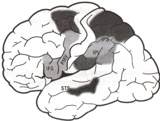
GÖRSEL 14: İnsan beyninde ayna nöron sistemi ile ilişkili temel bölgeler. Beynin birçok önemli alanını kaplayan bu sistem, kompleks motor ve sosyal davranışların öğrenilmesinde temel teşkil eder (Arch Neurol. 2009;66(5):557-560).
