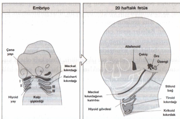
GÖRSEL 7: İnsan embriyo döneminde ve 20 haftalık fetüs döneminde gelişen temel yapılar.
