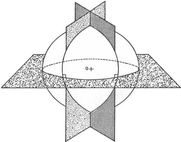
Şekil 3. Riemann
