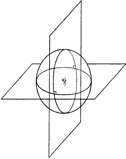
Şekil 2. Riemann
