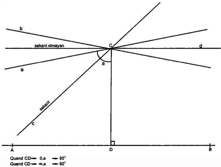
Şekil 1. Lobatchevski
