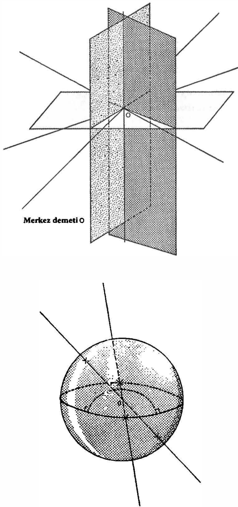
Şekil 1. Riemann
