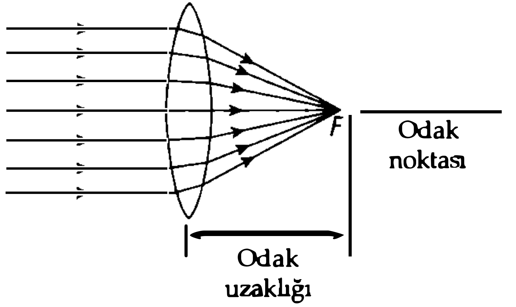
Şekil 4 a/b Yakınsak merceklerin işleyişi: a) yakındaki bir cismin görüntüsünün oluşumu. b) Uzaktaki ışınların odaklanması (Güneş).
