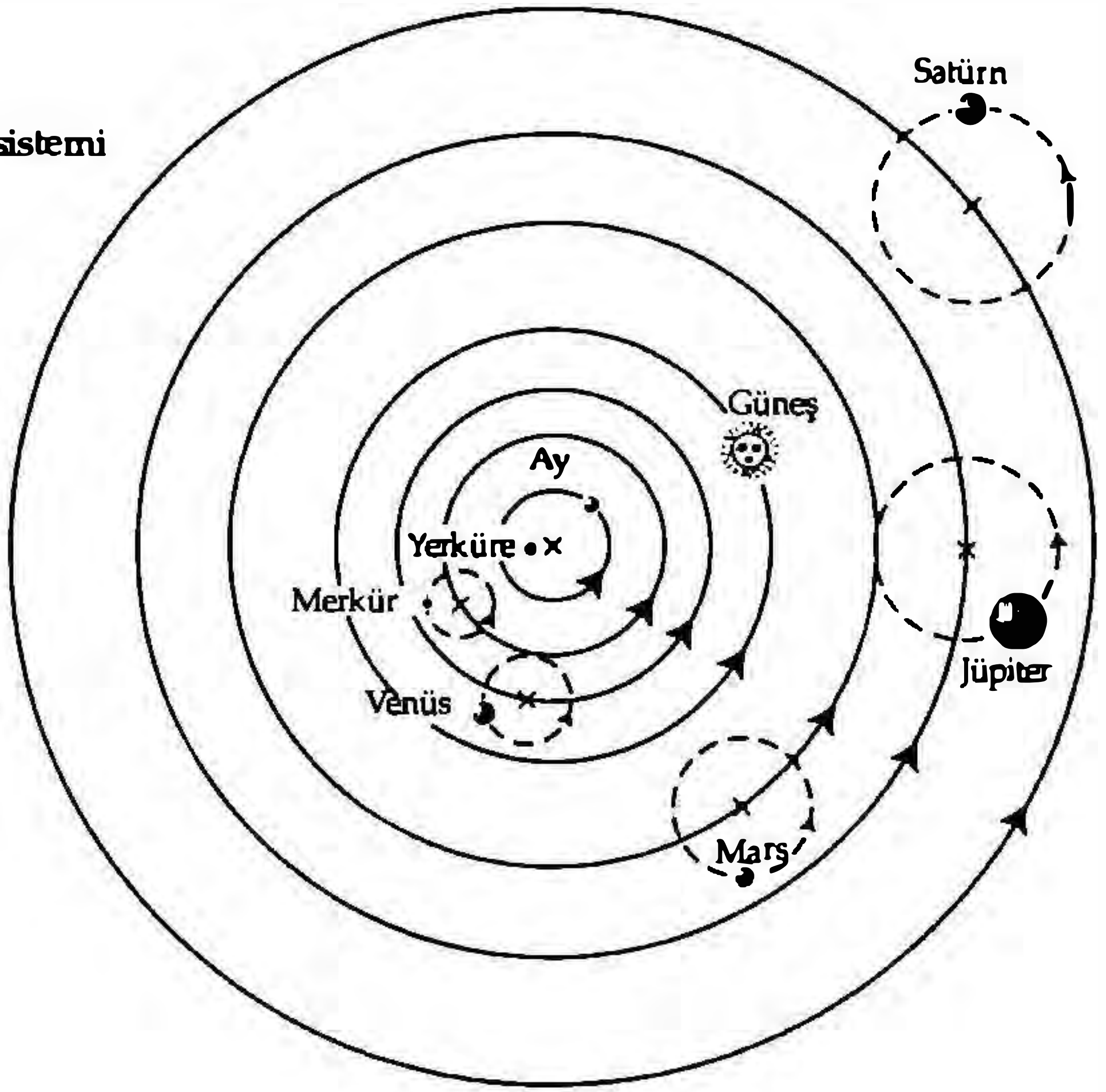
Tycho Brahe'nin Sistemi
