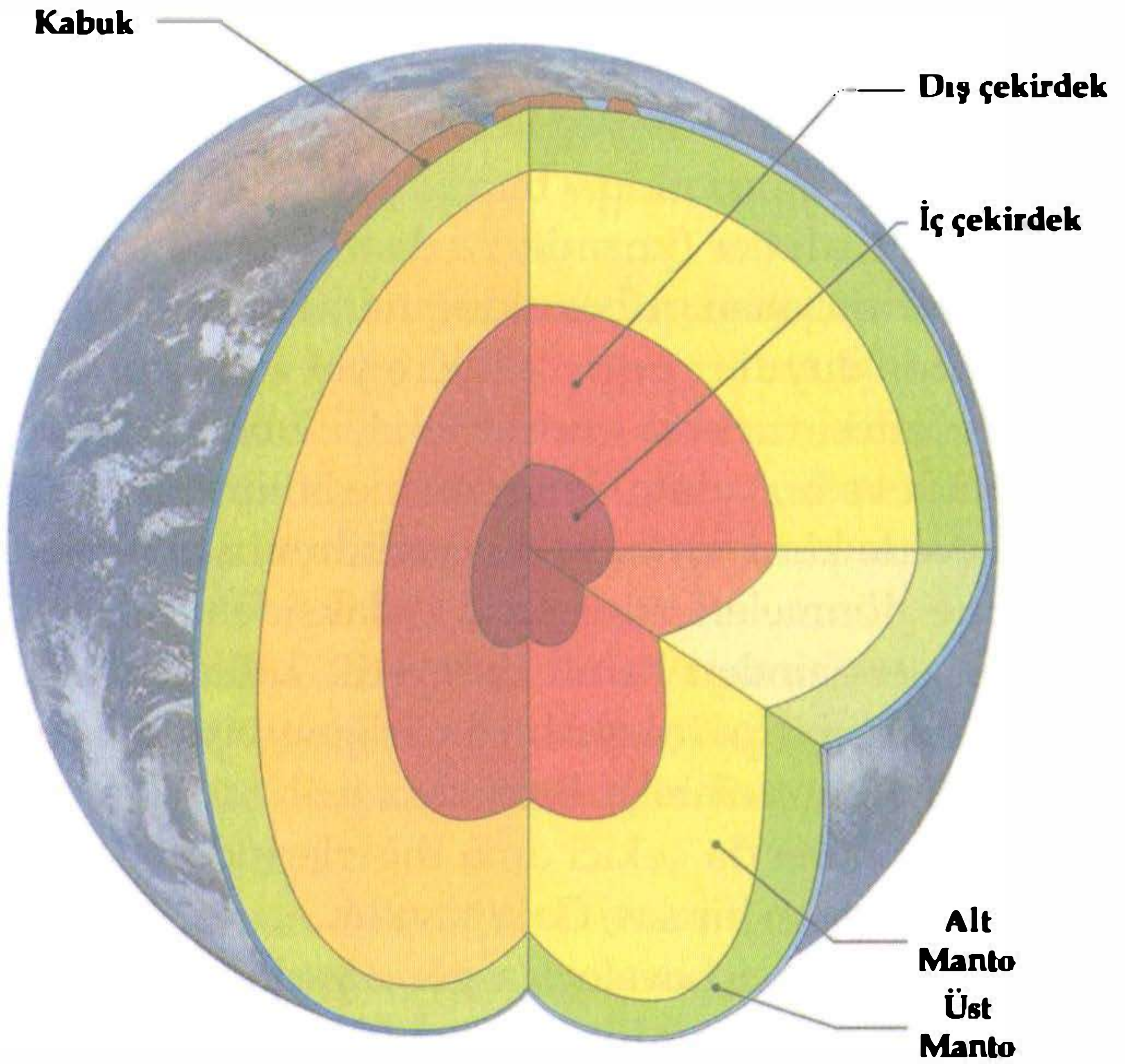
Şekil 11.5 Yerkürenin çeşitli katmanlarını gösteren kesit.
