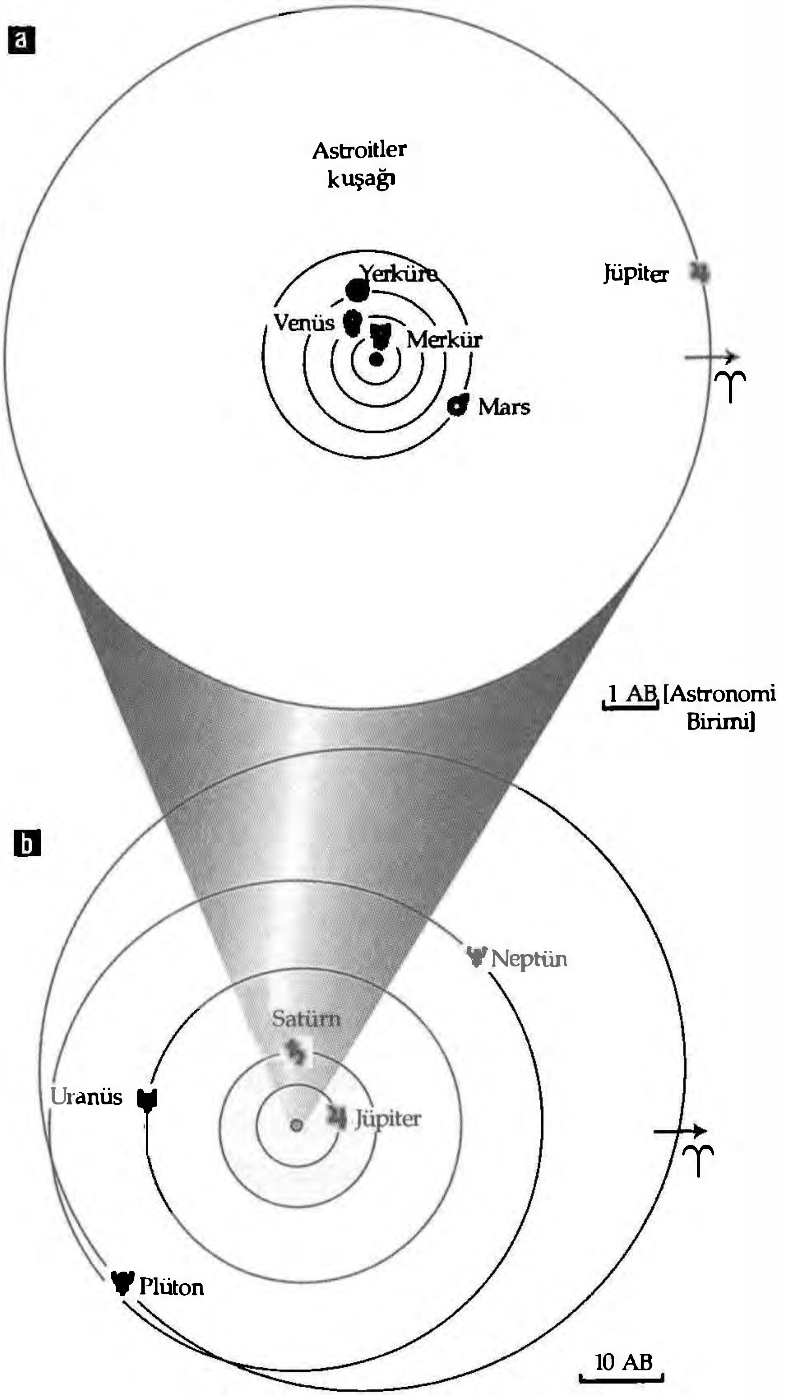
Şekil 4.6.b Kepler modelini gösteren şema.
