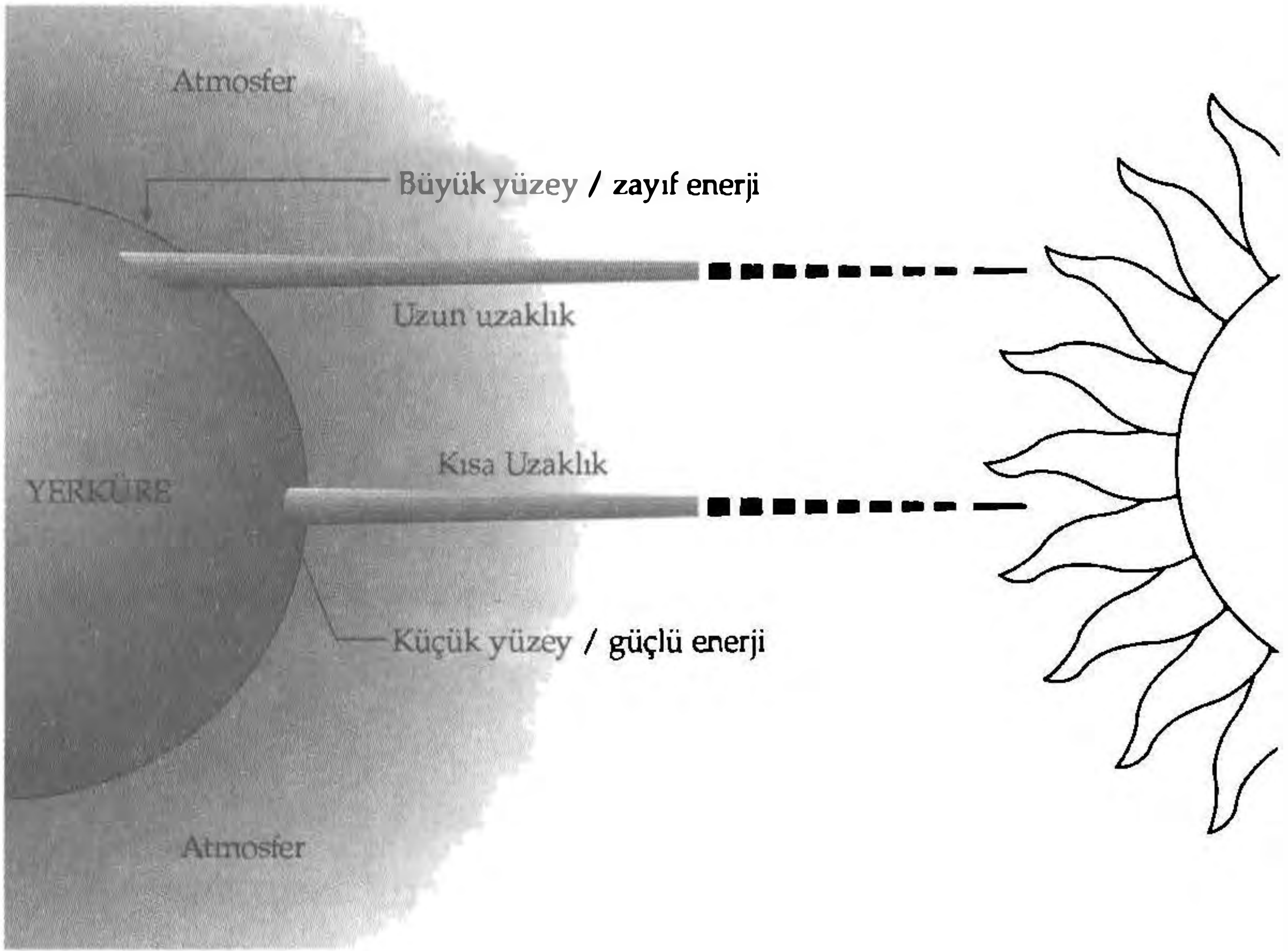
Şekil 11.3 Kutuplarda güneş almanın ekvatordakine göre nasıl daha az olduğunu gösteren şema.
