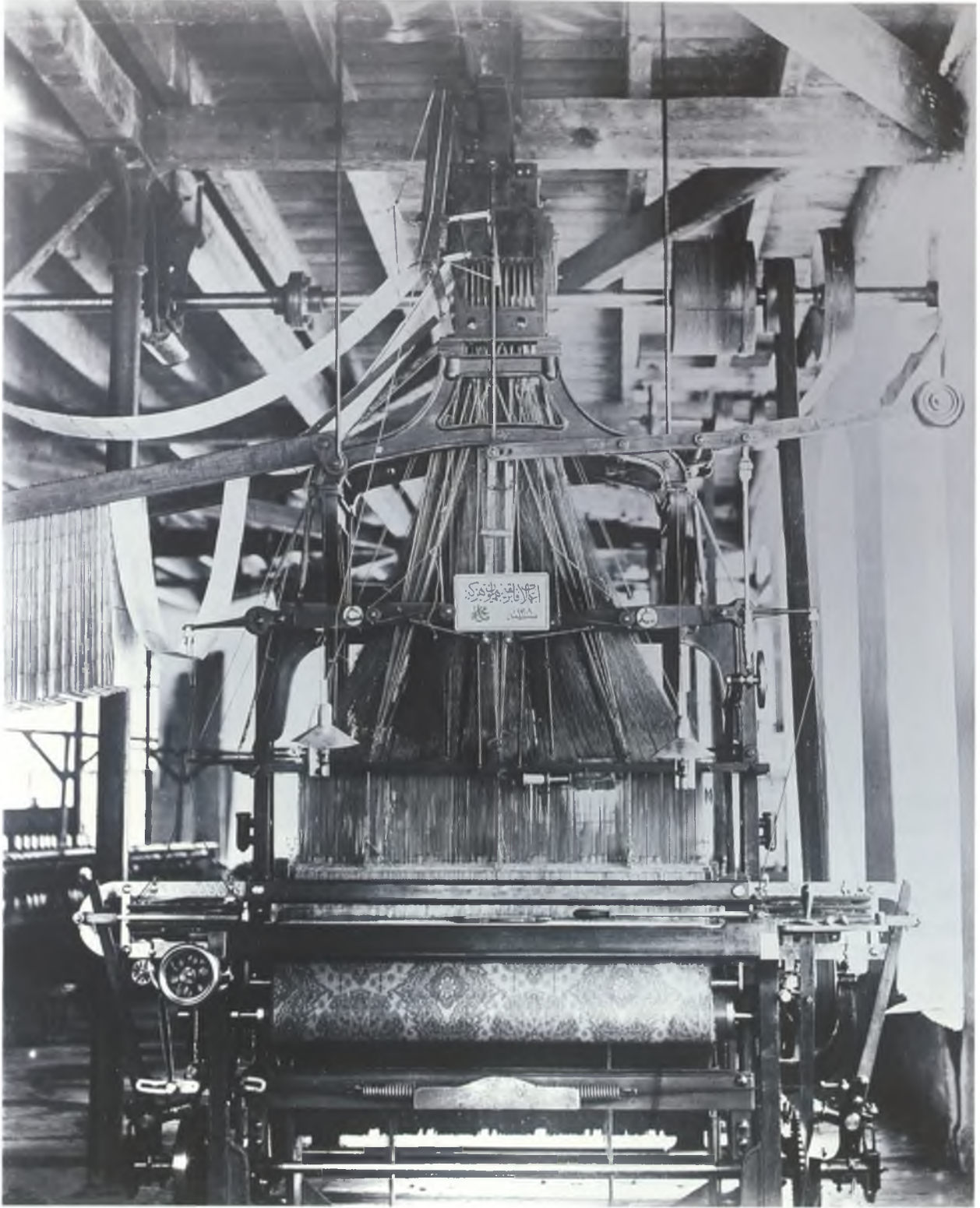
Hereke Fabrika-i Hümâyûnu'nda kullanılan jakar tezgâhı. IRCICA Fotoğraf Arşivi 90453-10.
