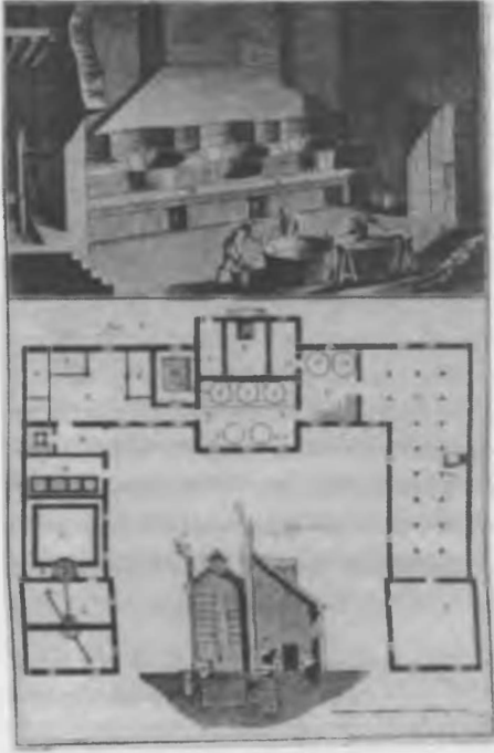
Şekil 18 Şeker imalathanesi ( Sucrerie ). Kaynak: Diderot ve d'Alembert, Encyclopédie , 18. cilt.
