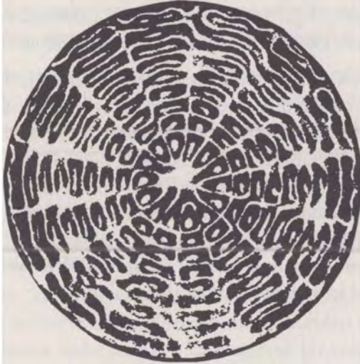
Kumla kaplı disk belli frekanslarda titreştirildiğinde oluşan şekil
