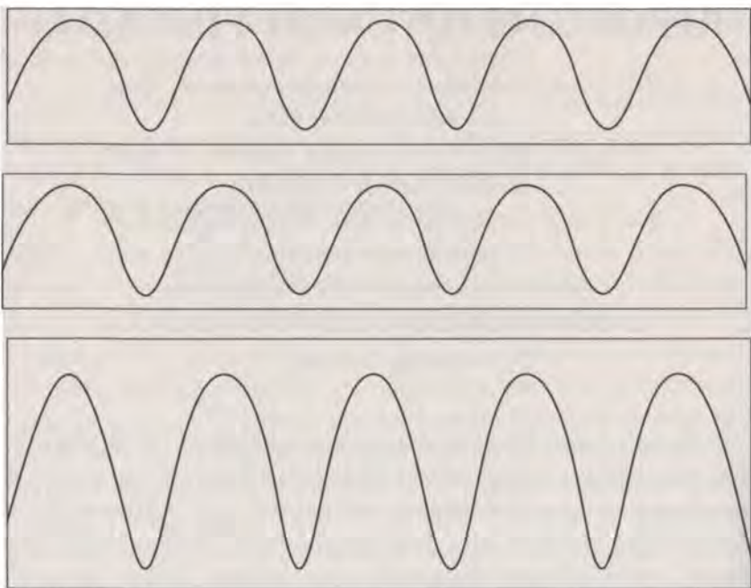
ŞEKİL 6.4 Ses dalgalarının yapıcı karışımı.
