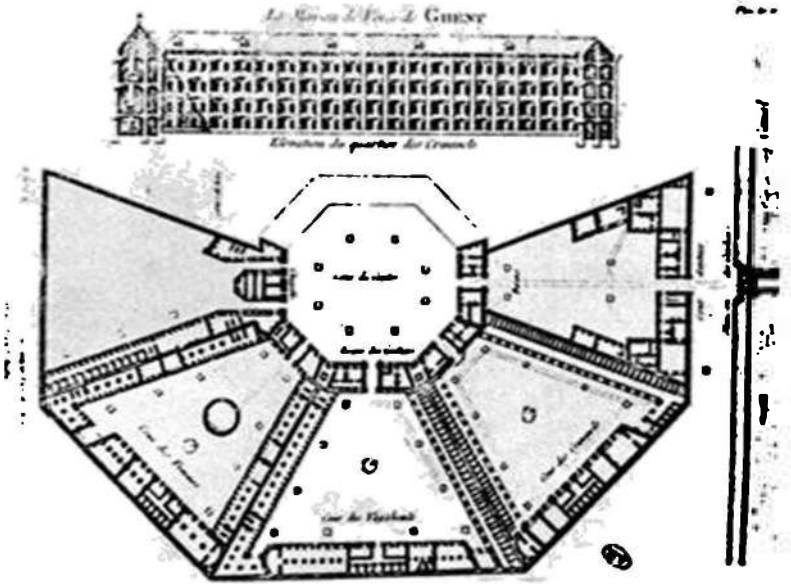
Gand güç evinin (hapishane) planı, 1773.
