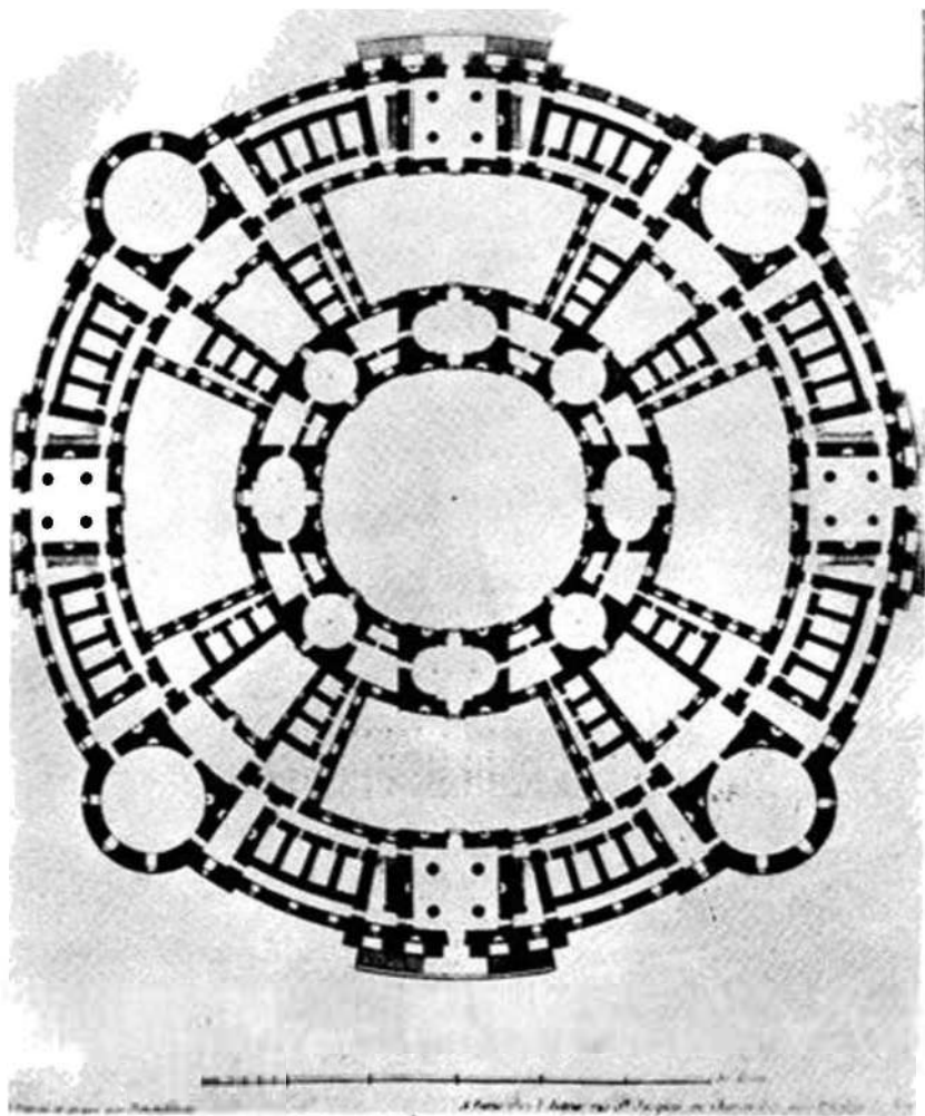
J. F. de Neufforge, Hapishane Projesinden.
