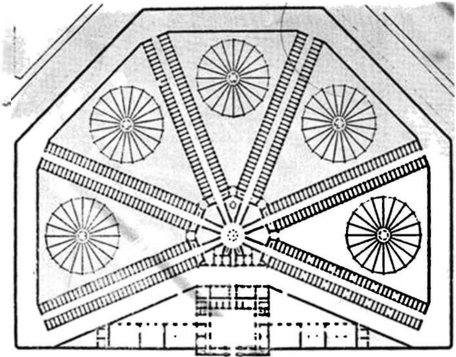
Mazas Hapishanesinin Planı.
