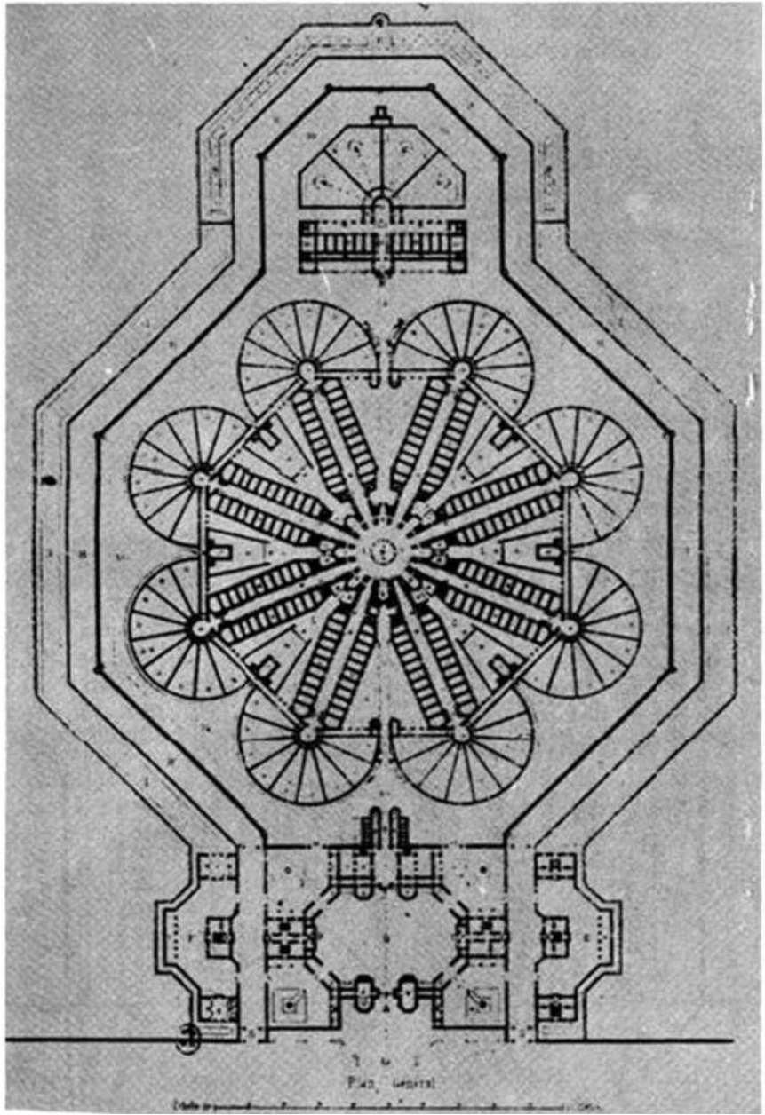
A. Blouet, 585 mahkûmluk hücreli hapishane projesi, 1843.
