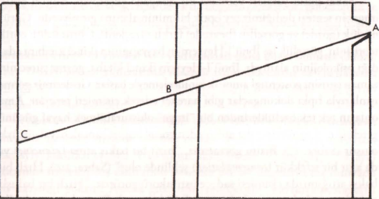
Res.38 İbnü'l- Heysem'in iki bölmeli düzeneğinin (bkz. Res. 37), Sezgin/ Neubauer'e (haz., 2003) dayanan çizimi
