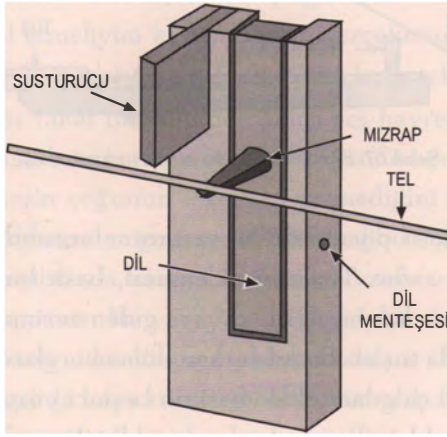
Şekil 68. Klavsende telleri çekme mekanizması.
