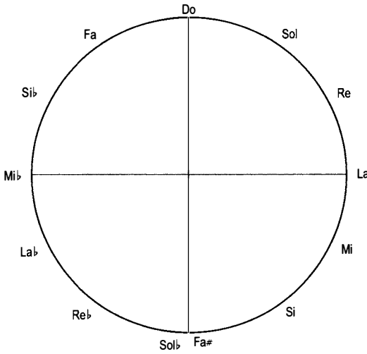
Şekil 60. Beşliler çemberi.
