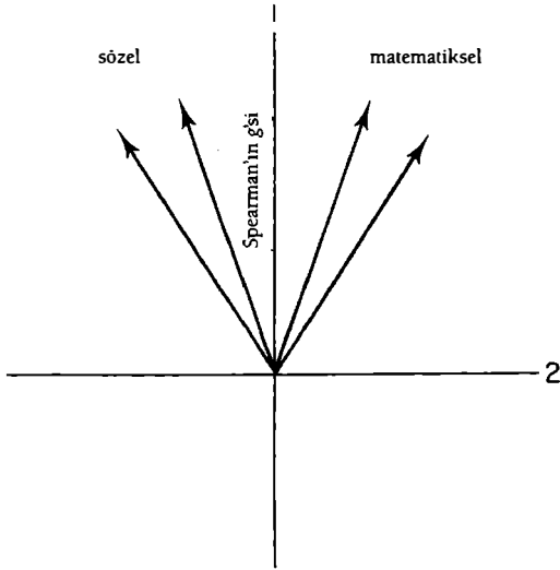
Şekil 6.6 Dört zeka testinin asal bileşen analizi. Bütün korelasyonlar yüksektir ve birinci asal bileşen, Spearman'ın g'si toplam korelasyonu açıklar. Ama sözel ve matematiksel beceriyi gösteren grup faktörleri bu analiz tarzında iyi çözülmez.
