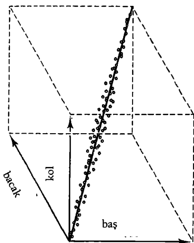
Şekil 6.3 Üç ölçüm için korelasyonları gösteren üç boyutlu bir grafik
