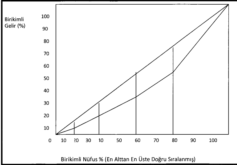
Şekil 1-5: Kesikli Dağılımda Gini Katsayısı Hesabında Kullanılan Alanlar
