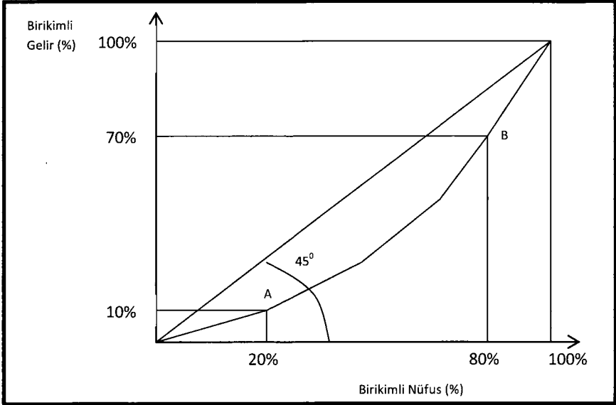
Şekil 1-3: Bir Gelir Dağılımına Ait Lorenz Eğrisi
