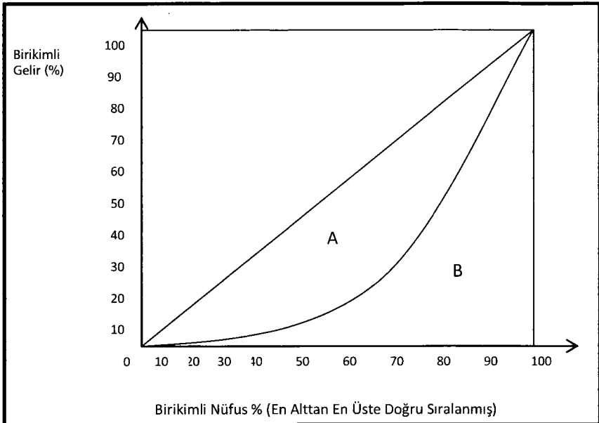
Şekil 1-4: Lorenz Eğrisinden Gini Katsayısının Hesaplanması
