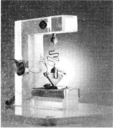
Bell Labs'te ilk transistör.
