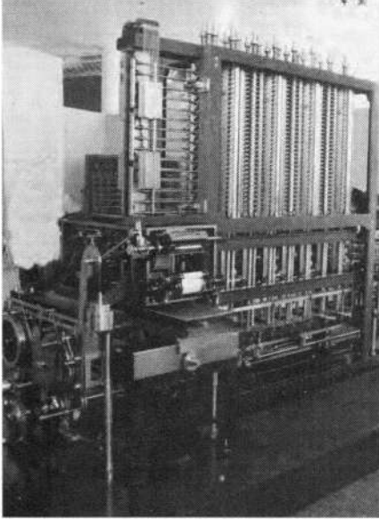
Fark Makinesi'nin bir kopyası.
