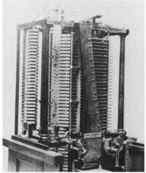
Analitik Makine'nin bir kopyası.
