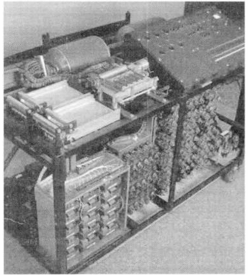
Atanasoff'un bilgisayarının rekonstrüksiyonu.
